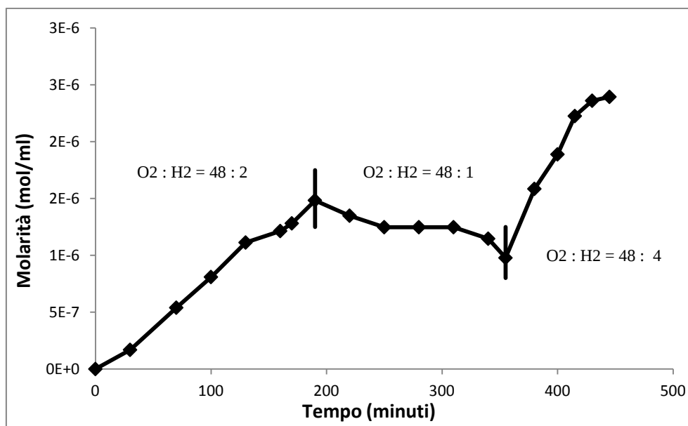
Figura 3.4: Andamento della produzione di \text{H}_2\text{O}_2 nel tempo, espressa in moli/ml.
