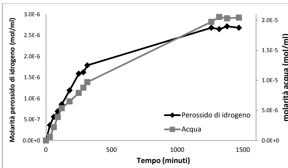
Figura 5.7: Andamento della produzione di perossido di idrogeno nel tempo e di acqua, espressi in moli/ml.
