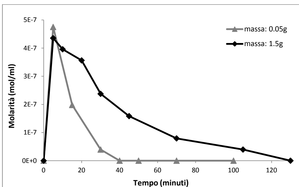
Figura 5.3: Rappresentazione dell'andamento della produzione di perossido di idrogeno nel tempo, espressa in moli/ml.
