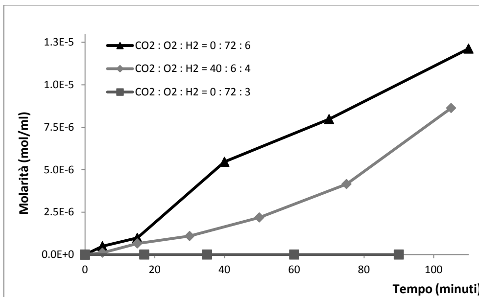
Figura 3.2: Rappresentazione dell'andamento della produzione di H_2O nel tempo, espressa in moli/ml.
