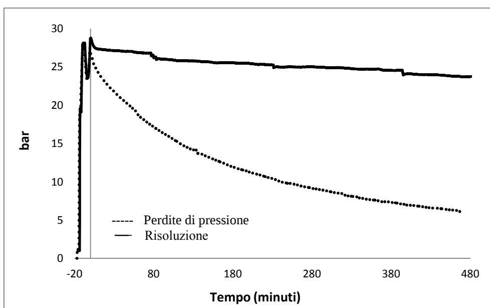
Figura 4.6: Rappresentazione dell'andamento della pressione interna al reattore prima e dopo aver determinato le perdite di pressione.
