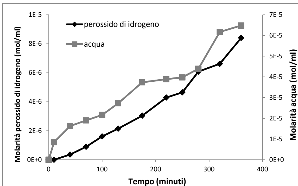
Figura 3.3: Confronto tra la produzione di H_2O_2 e H_2O nel tempo.
