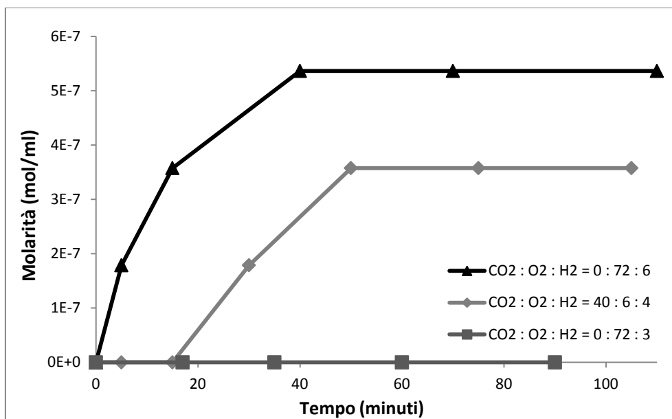
Figura 3.1: Rappresentazione dell'andamento della produzione di H_2O_2 nel tempo, espressa in moli/ml.
