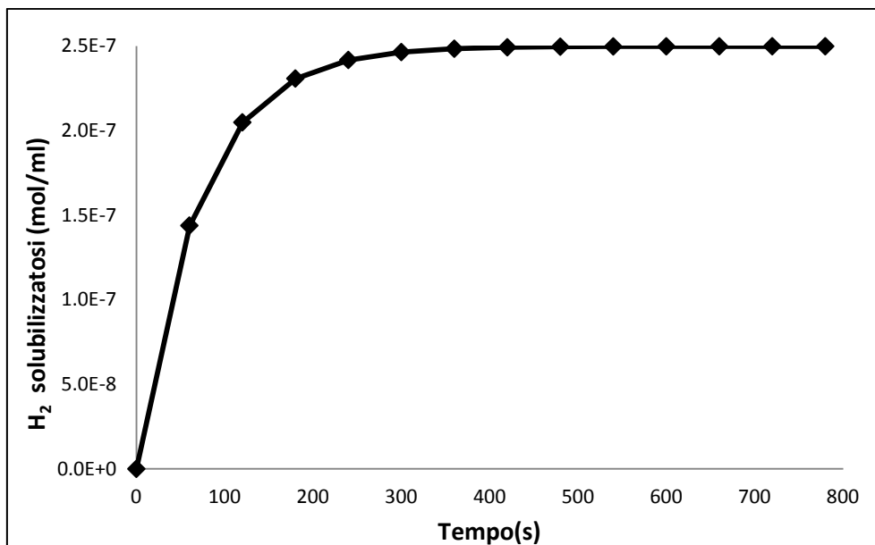
Figura 2.4: Rappresentazione della quantità di idrogeno solubilizzatosi nel metanolo al variare del tempo.
