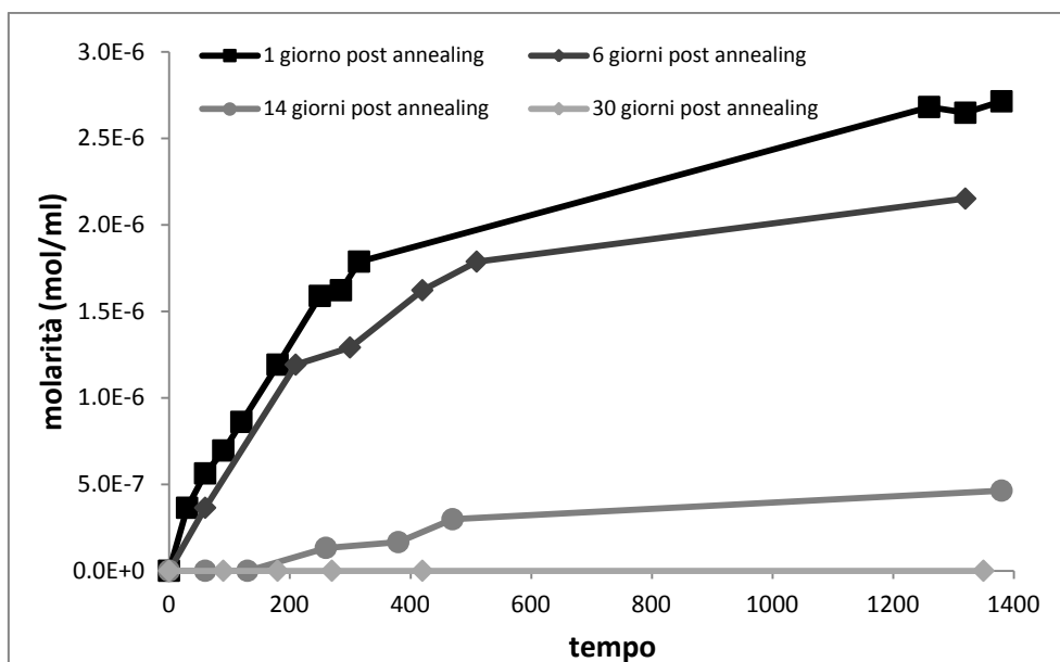
Figura 5.9: Rappresentazione dell'andamento della produzione di perossido di idrogeno nel tempo, espressa in mol/ml.
