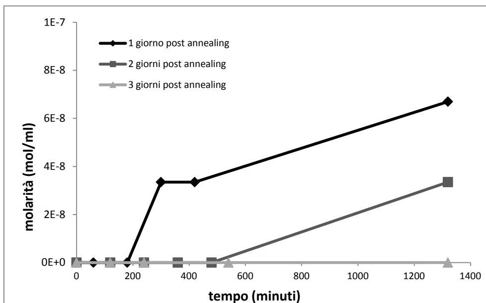
Figura 5.10: Rappresentazione dell'andamento della produzione di perossido di idrogeno nel tempo, espressa in mol/ml.
