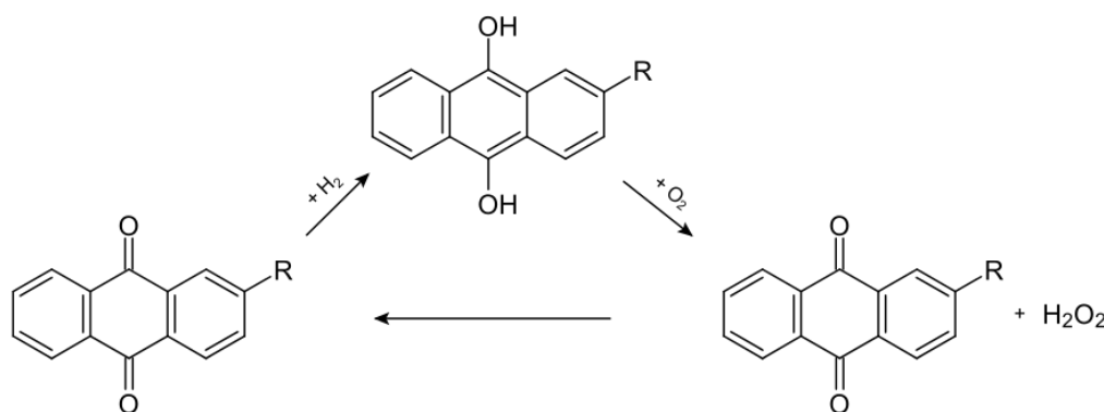
Figura 1.1: Rappresentazione del ciclo della sintesi tramite antrachinone.
