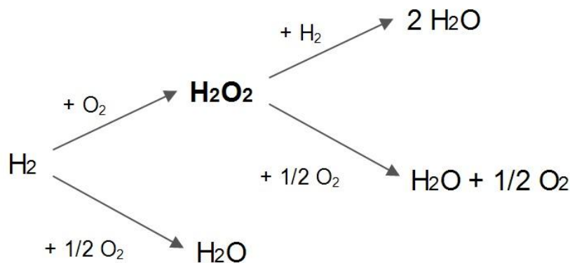
Figura 1.3: Rappresentazione schematica delle reazioni coinvolte.
