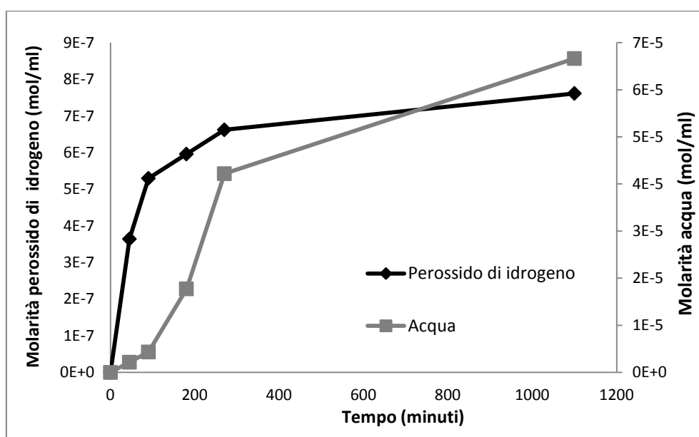
Figura 5.4: Rappresentazione dell'andamento della produzione nel tempo di perossido di idrogeno e di acqua.
