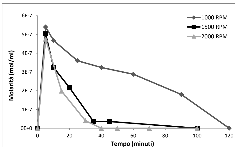
Figura 5.2: Rappresentazione dell'andamento della produzione di perossido di idrogeno nel tempo, espressa in moli/ml.
