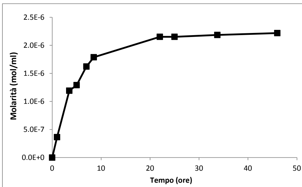
Figura 5.8: Rappresentazione dell'andamento della produzione di perossido di idrogeno nel tempo, espressa in mol/ml.
