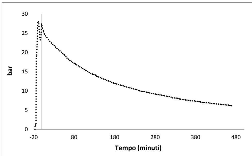
Figura 4.5: Rappresentazione dell'andamento della pressione interna al reattore durante la prima prova sperimentale.
