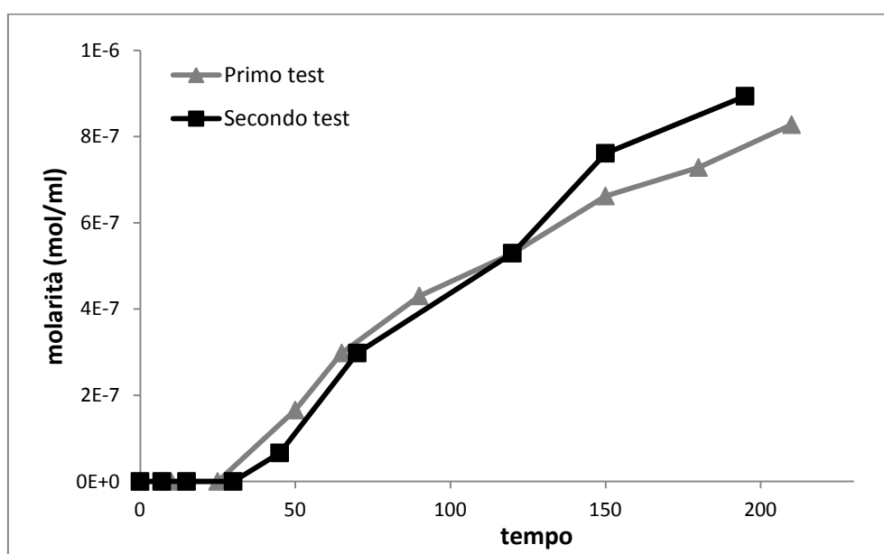
Figura 5.6: Rappresentazione dei profili di produzione per le due prove.
