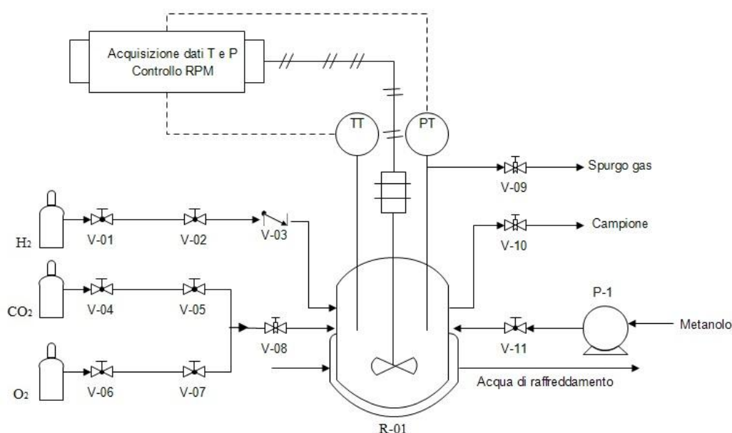
Figura 4.2: Rappresentazione schematica dell'apparato sperimentale.
