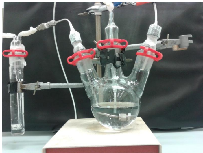
Figura2.1: Rappresentazione dell'apparato sperimentale.
