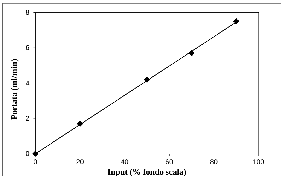
Figura 2.5: Retta di taratura per il mass flow controller MF-12, impiegato per il controllo della portata di idrogeno. In ascissa vi sono i valori di input, espressi in percentuale di fondo scala, in ordinata è riportata la portata erogabile.
