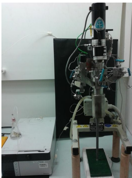
Figura 4.1: Rappresentazione dell'apparato sperimentale.
