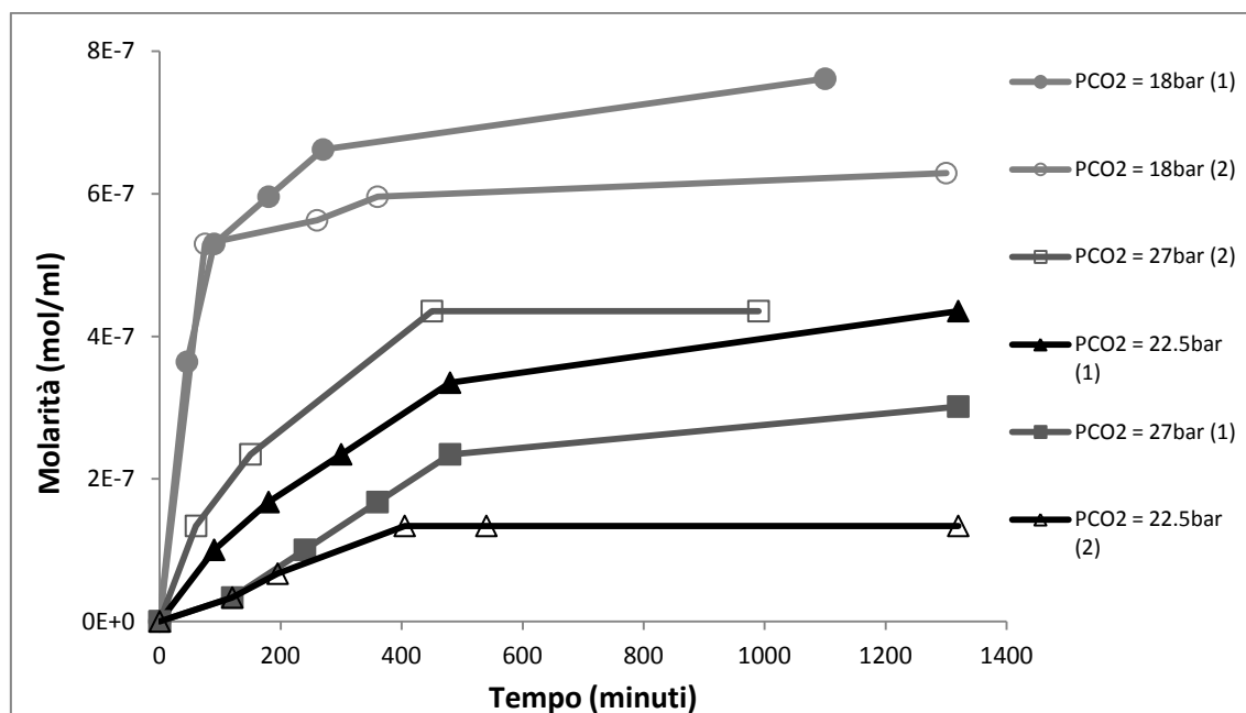
Figura 5.5: Rappresentazione dell'andamento della produzione di perossido di idrogeno nel tempo, espressa in moli/ml.
