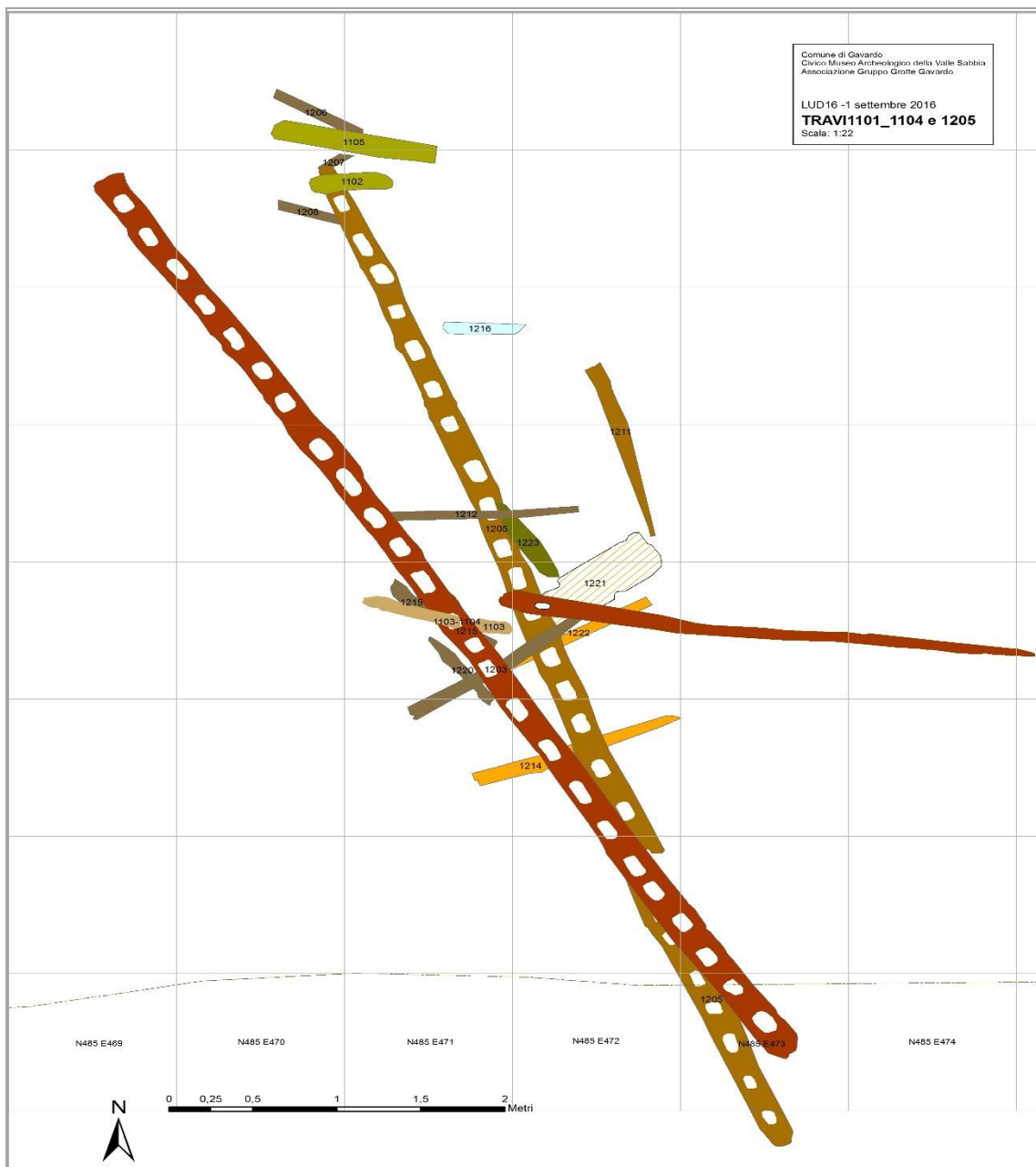
Fig. 17 le due travi di quasi 8 m ciascuna con 25 fori quadrangolari (ripresa e modificata da Baioni, Mangani, Martinelli, 2021).
