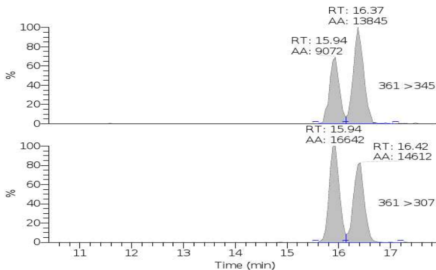
Figura 5: Cromatogrammi ottenuti da campioni di urina bianchi addizionati con 2,5 ng/ml di betametasone (tempo di ritenzione 15,9 minuti) e desametasone (tempo di ritenzione 16,4 minuti).
