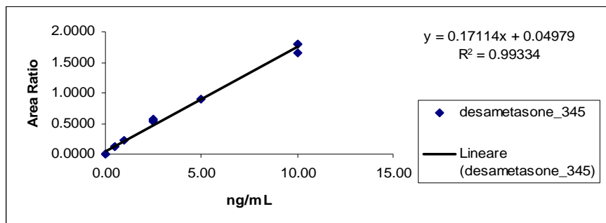
Figura 6: Retta di calibrazione in matrice.
