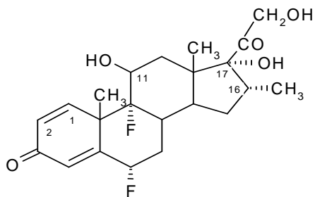
Flumetasone
