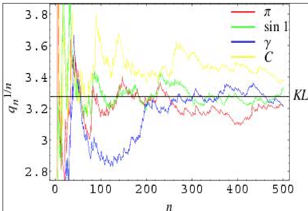
Figura 4: Grafico dell'andamento della media geometrica dei denominatori delle prime 500 convergenti nello sviluppo in frazioni continue di alcuni numeri reali.
