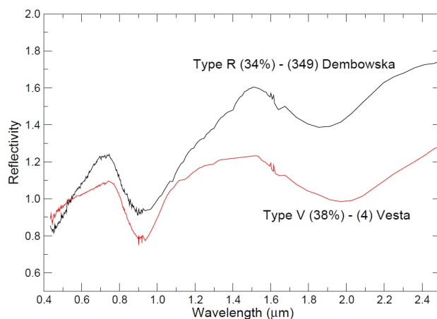
Figura 2.2: Esempio di spettri di tipo V e R. Gli spettri sono normalizzati a 0.55 \mu\text{m} . Tra parentesi è riportato il range di albedo in percentuale. (Magrin, 2006)
