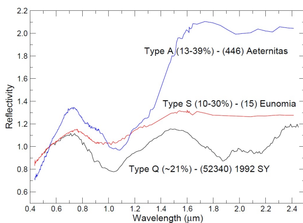
Figura 2.1: Esempio di spettri di tipo Q, S e A. Gli spettri sono normalizzati a 0.55 \mu\text{m} . Tra parentesi è riportato il range di albedo in percentuale. (Magrin, 2006)
