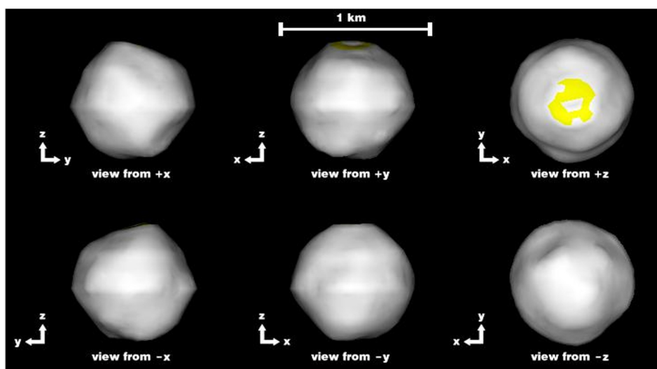
Figura 4.9: Vista degli assi principali del modello della forma del primario. Il modello ha 1000 vertici e 1996 facets triangolari. La risoluzione efficace è \sim 50 m . Le regioni in giallo indicano regioni in cui l'angolo di incidenza e di scattering è > 60^\circ . (Naidu et al., 2020)
