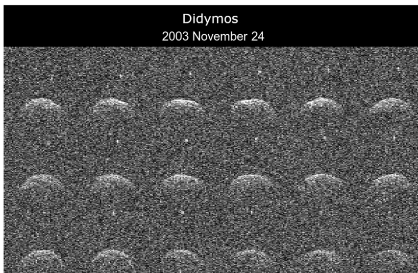
Figura 4.8: Immagini delay-Doppler ottenute con il telescopio di Arecibo il 24 novembre 2003 tra le 03:15 e le 05:09 UTC. Ogni immagine è la somma di tre pose, durante le quali il primario ha ruotato di 14^\circ . La risoluzione dell'immagine è di 0.1 \mu s \times 0.3 Hz . (Naidu et al., 2020)
