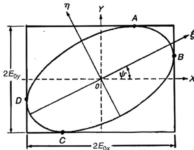
Figura 1.2: Ellisse di polarizzazione
