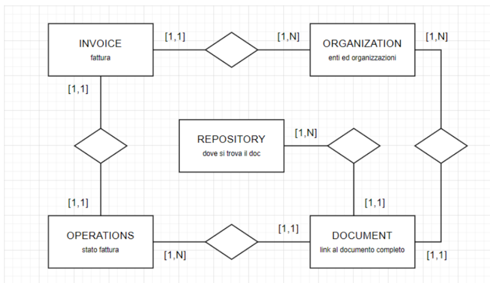
Figura 5.1: Diagramma ER per la sezione semplificata di InvoiceChannel
