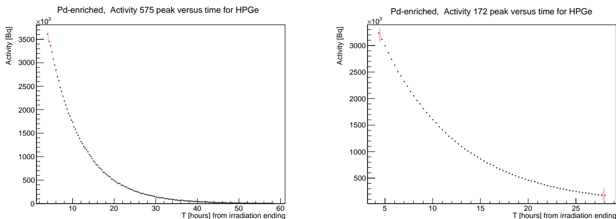
Figura 3.14: Andamento attività delle righe 575 keV e 172 keV di ^{111m}Pd in funzione del tempo
