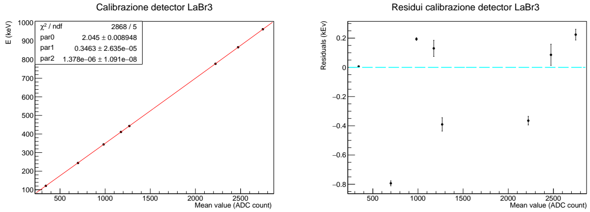
Figura 3.2: Plot di calibrazione in energia con annessi residui per LaBr 3
