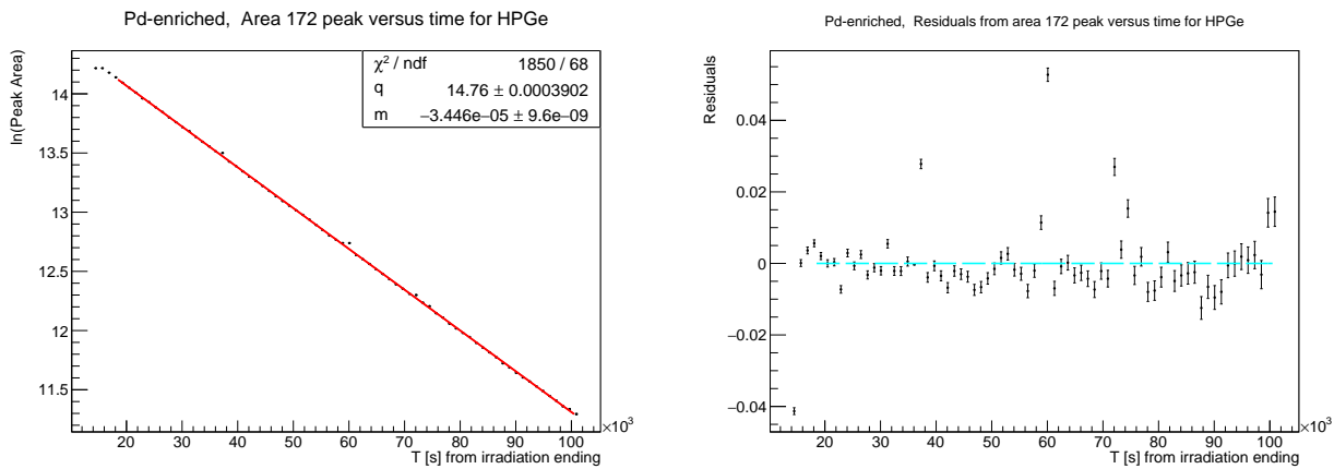
Figura 3.13: Fit linearizzato per la stima del tempo di dimezzamento di ^{111m}Pd , picco 172 keV
