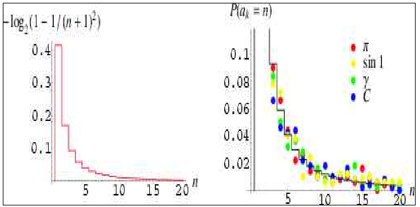
Figura 3: Distribuzione di probalilita' di Gauss dei primi 500 termini nello sviluppo in frazioni continue di alcuni numeri reali
