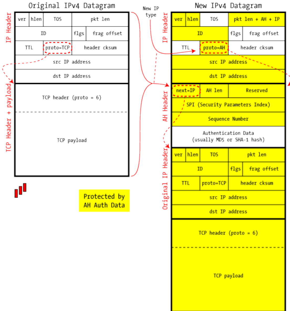
Figura 1.5: Inserimento di AH in un datagramma IP in modalità tunnel. L'uso di TCP nel payload IP è puramente esemplificativo. In giallo i componenti la cui integrità è protetta da AH.[2]
