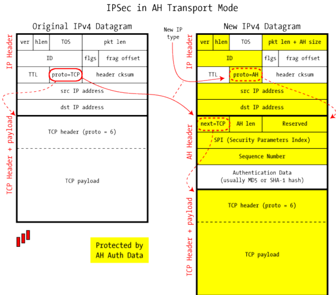
Figura 1.4: Inserimento di AH in un datagramma IP in modalità transport. L'utilizzo di TCP nel payload IP è puramente esemplificativo. In giallo i componenti la cui integrità è protetta da AH.[2]
