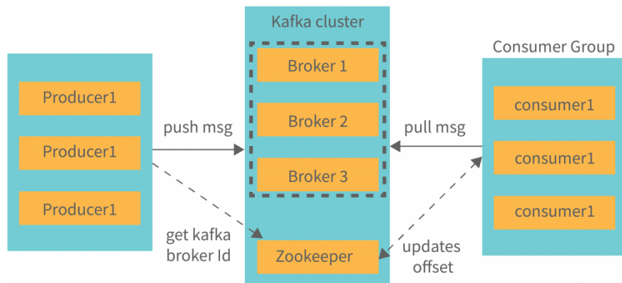
Figura 3.2: Architettura di Apache Kafka
