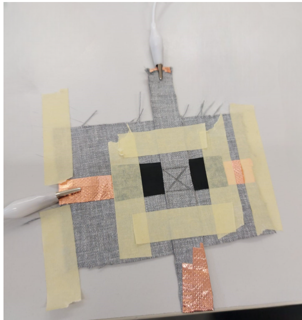
Figura 2.2: Setup per il metodo di stima della funzione
