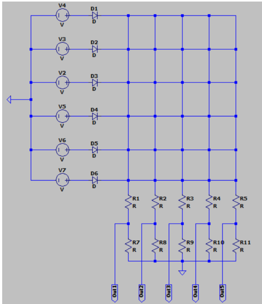
Figura 3.1: Schema del circuito creato utilizzando LTspice [13].
