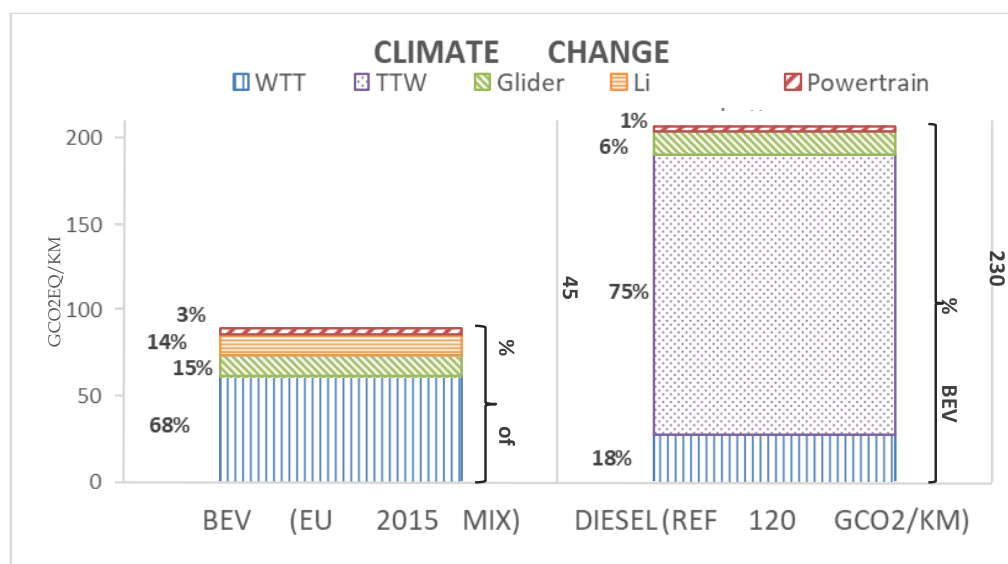
Figura 17 – Confronto tra impatti climalteranti di ICEV e BEV suddivisi pe fasi.
