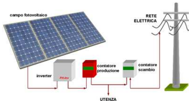
Figura 12: Impianto fotovoltaico
