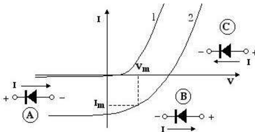
Figura 8: Caratteristica del fotodiode
