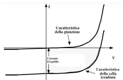
Figura 9: Caratteristica della cella al buio e della cella irradiata
