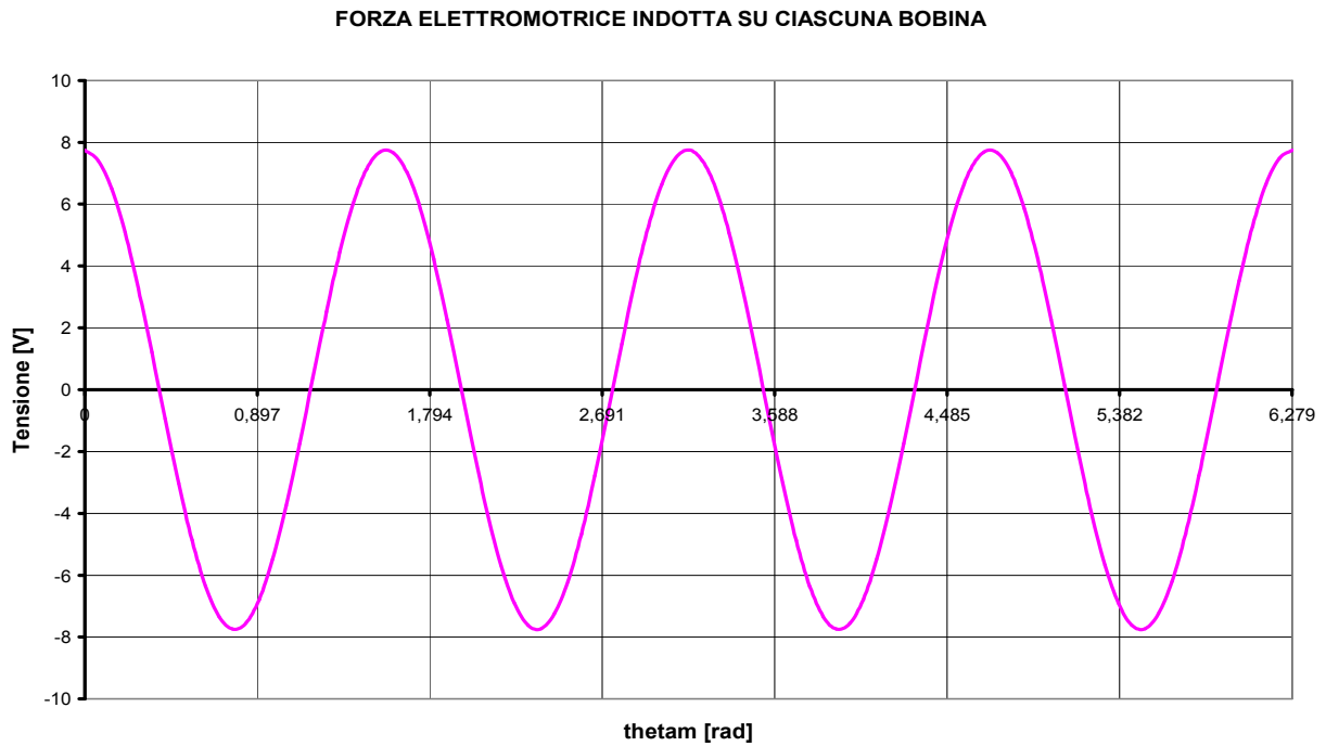
Fig. 2.91: Forza elettromotrice generata a carico in regime continuo (modello 3)
