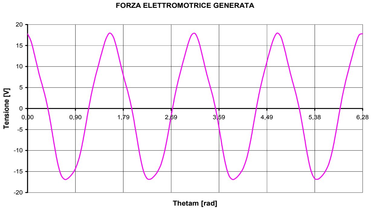
Fig. 7.26: Forza elettromotrice generata per \omega_m = 170 [rad/s] in regime sinusoidale
