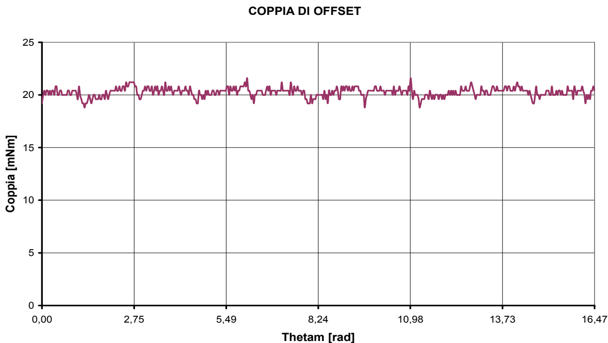
Fig. 7.48: Coppia di offset misurata con torsionometro meccanico per \omega_m = 170 [rad/s]
