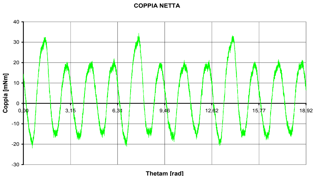
Fig. 5.34: Coppia al netto dell' offset per \omega_m = 18.54 [rad/s] in regime continuo
