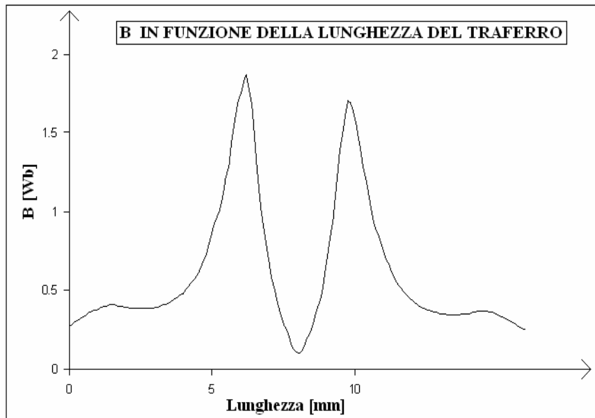
Fig. 7.19: Campo magnetico lungo il traferro a regime sinusoidale
