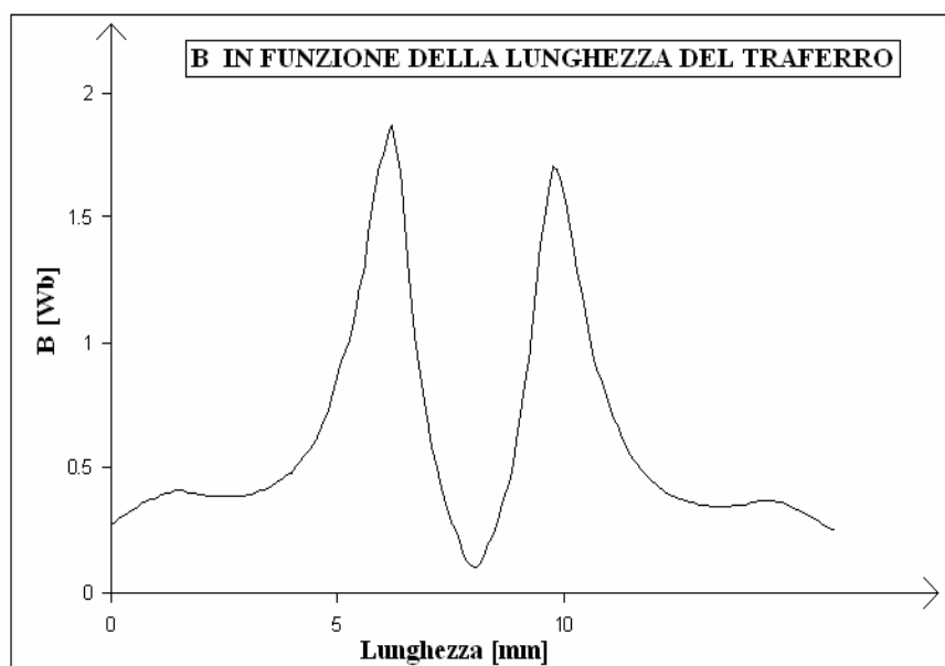
Fig. 7.18: Campo d' induzione magnetica lungo il traferro a regime sinusoidale
