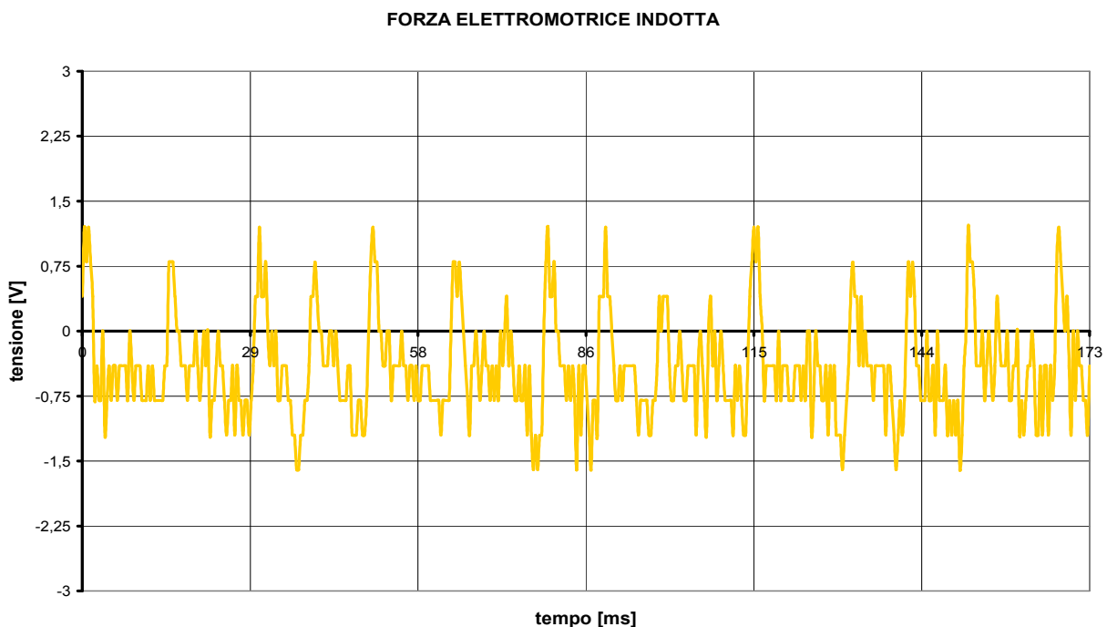
Fig. 7.41: Forza elettromotrice generata a vuoto per \omega_m = 10.74 [rad/s]
