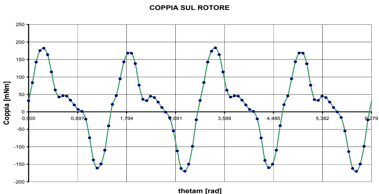
Fig. 7.54: Coppia in regime sinusoidale ottenuta con software di simulazione FEMM
