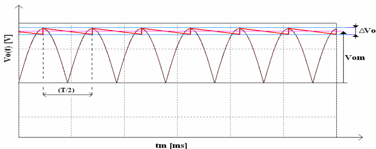
Fig. 4.5: Forma d' onda idealizzata della tensione sul carico
