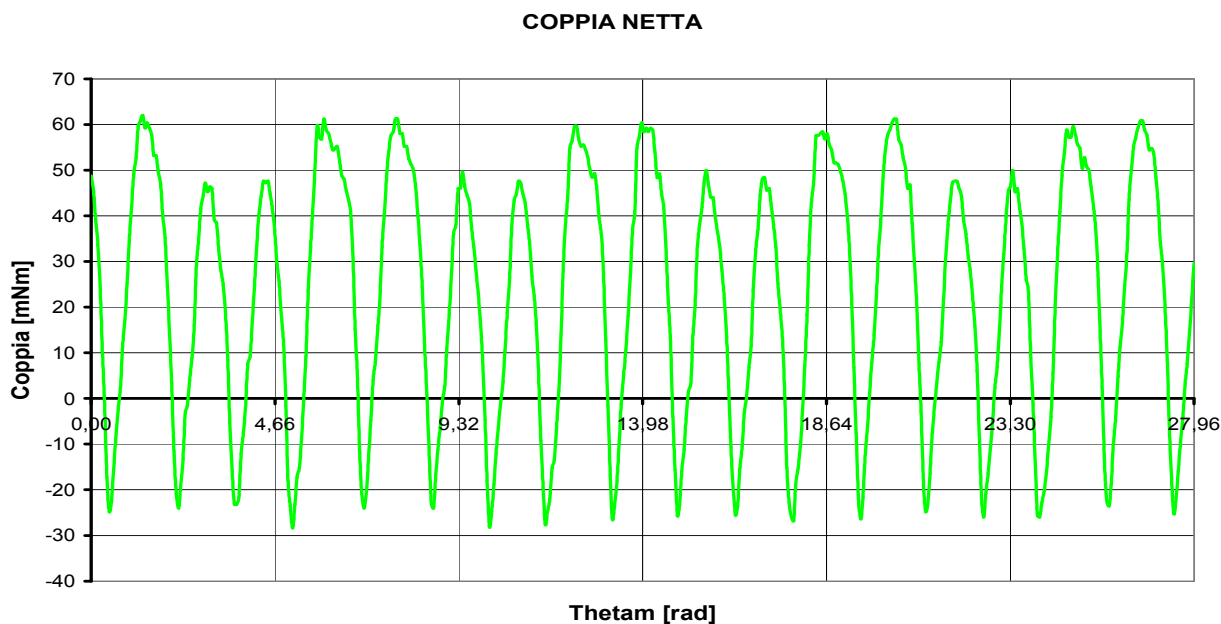
Fig. 7.53: Coppia misurata con torsionometro in regime sinusoidale per \omega_m = 30 [rad/s]
