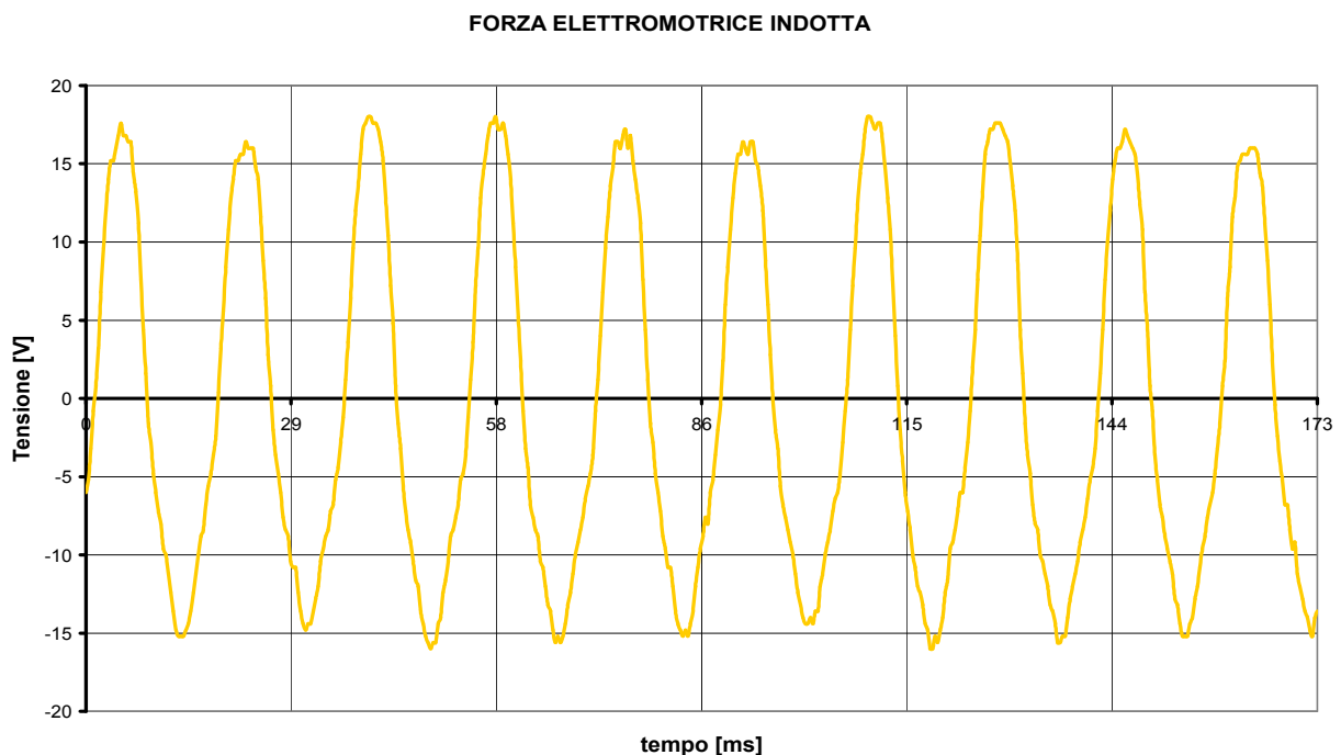
Fig. 7.36: Tensione generata a vuoto dal generatore bipolare per \omega_m = 170 [rad/s]
