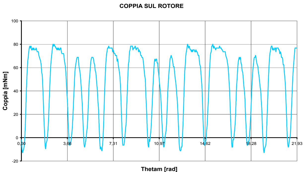
Fig. 7.42: Coppia a vuoto misurata con torsionmetro meccanico per \omega_m = 10.74 [rad/s]
