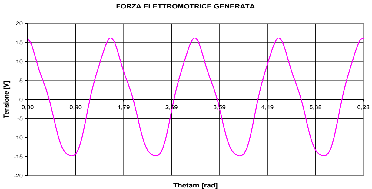
Fig. 7.15: Forza elettromotrice generata a vuoto dal generatore bipolare
