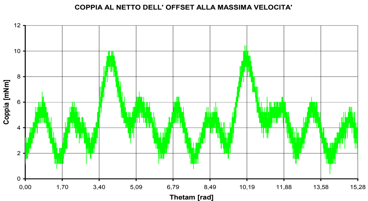
Fig. 5.20: Coppia netta a vuoto misurata con torsionometro meccanico per \omega_m = 154.12 [rad/s]
