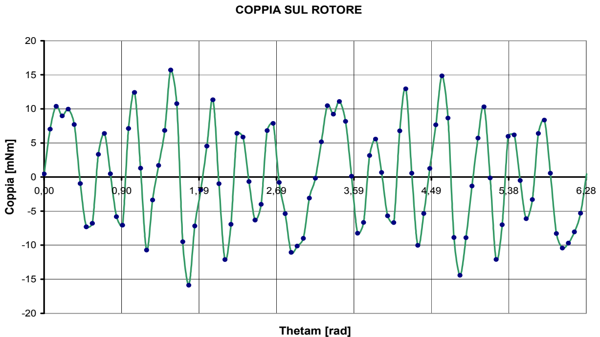
Fig. 5.21: Coppia a vuoto simulata mediante software FEMM per \omega_m = 154.12 [rad/s]
