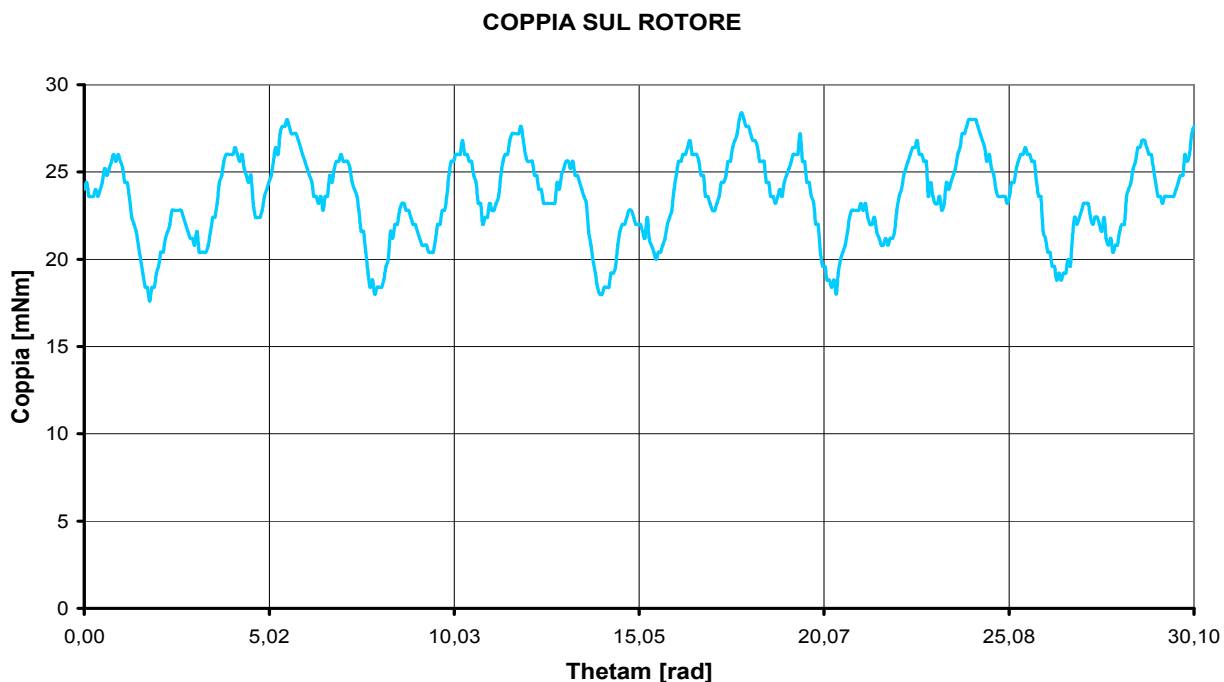
Fig. 7.61: Coppia misurata con torsionometro in regime continuo per \omega_m = 170 [rad/s]
