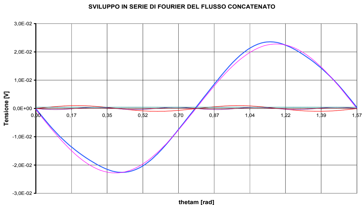
Fig. 2.90: Sviluppo in serie di Fourier del flusso concatenato: modello 3 in regime continuo
