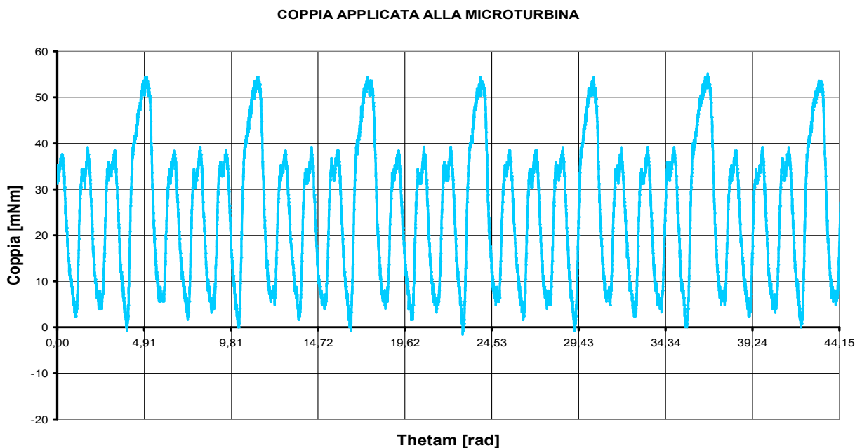
Fig. 5.13: Coppia a vuoto misurata con torsionmetro meccanico per \Omega_m = 10.74 [rad/s]
