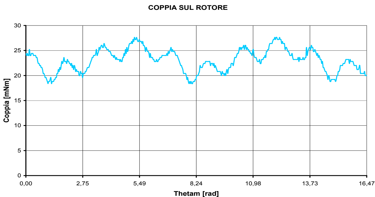
Fig. 7.47: Coppia a vuoto misurata con torsionometro meccanico per \omega_m = 170 [rad/s]
