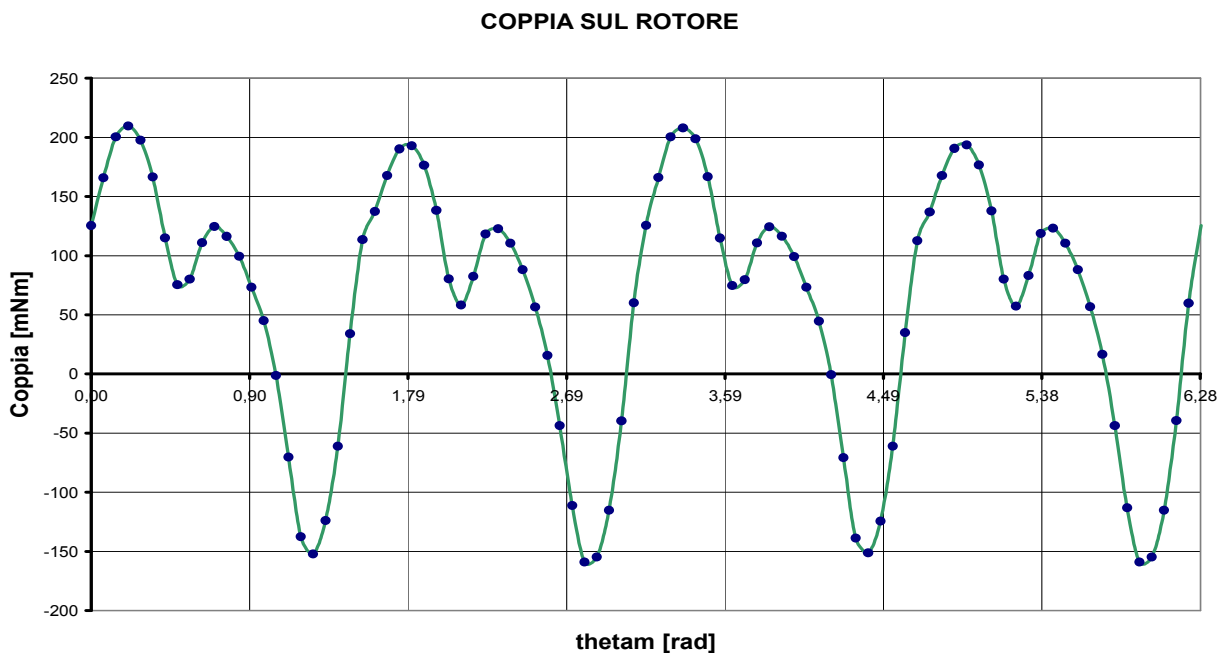
Fig. 7.58: Coppia in regime sinusoidale ottenuta con software di simulazione FEMM
