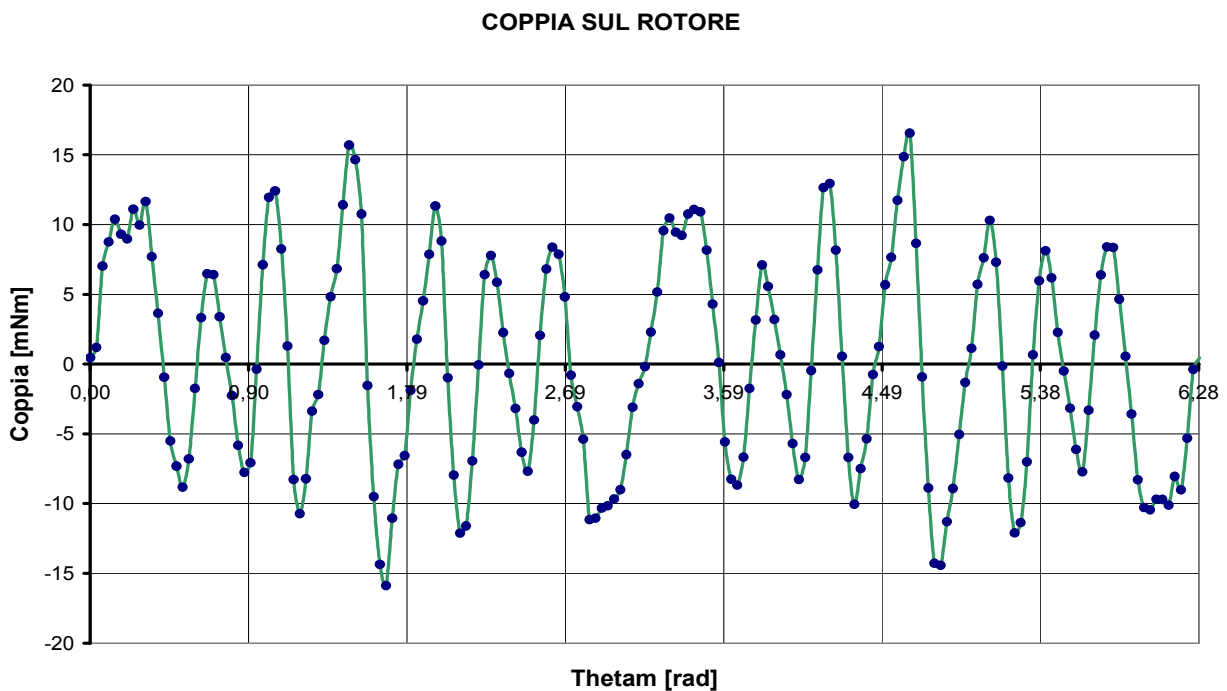
Fig. 2.69: Coppia sul rotore in funzione di \theta_m (modello definitivo a vuoto)
