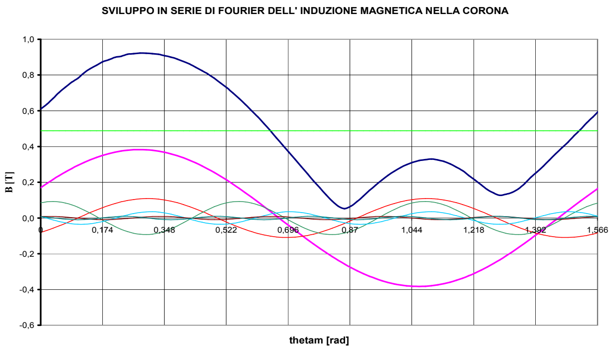
Fig. 6.6: Sviluppo in serie di Fourier di |\dot{B}| in funzione di \theta_m
