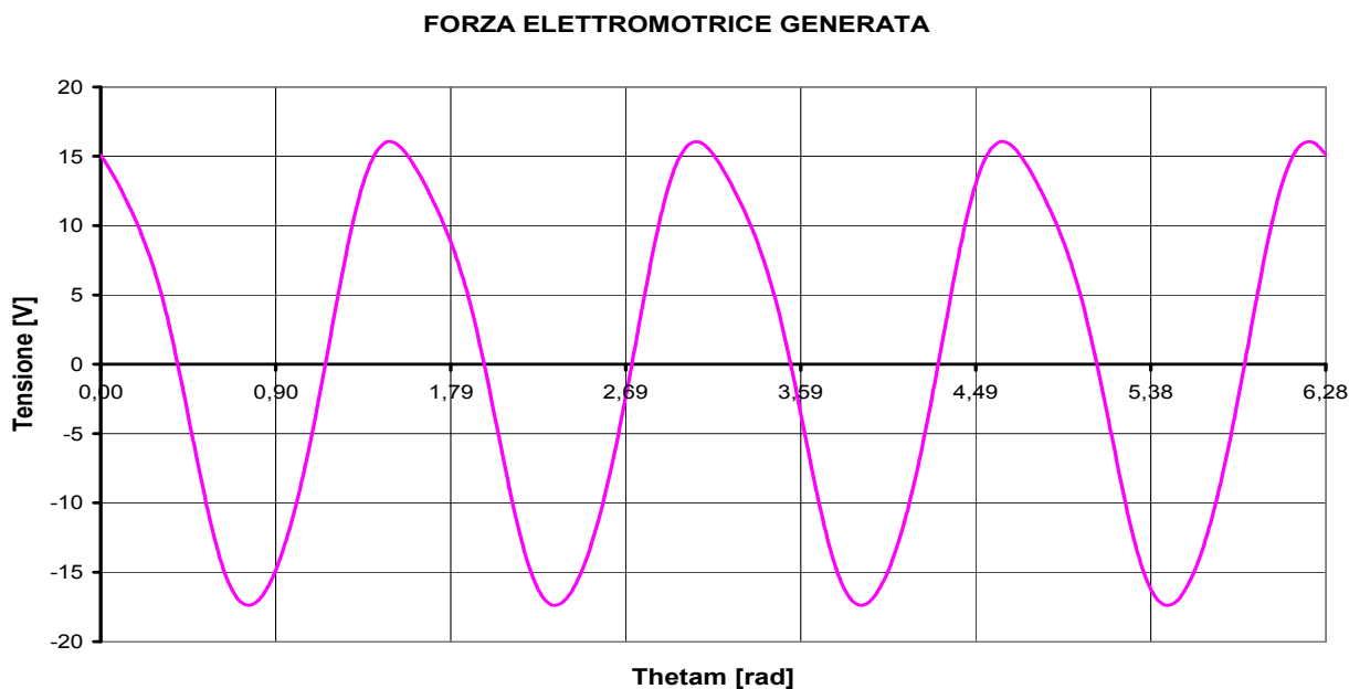
Fig. 7.32: Forza elettromotrice generata per \omega_m = 170 [rad/s] in continuo
