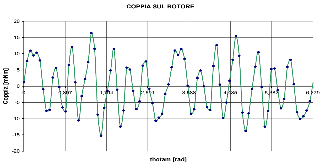
Fig. 5.39: Coppia ottenuta dalla simulazione per \omega_m = 151.31 [rad/s] in regime continuo
