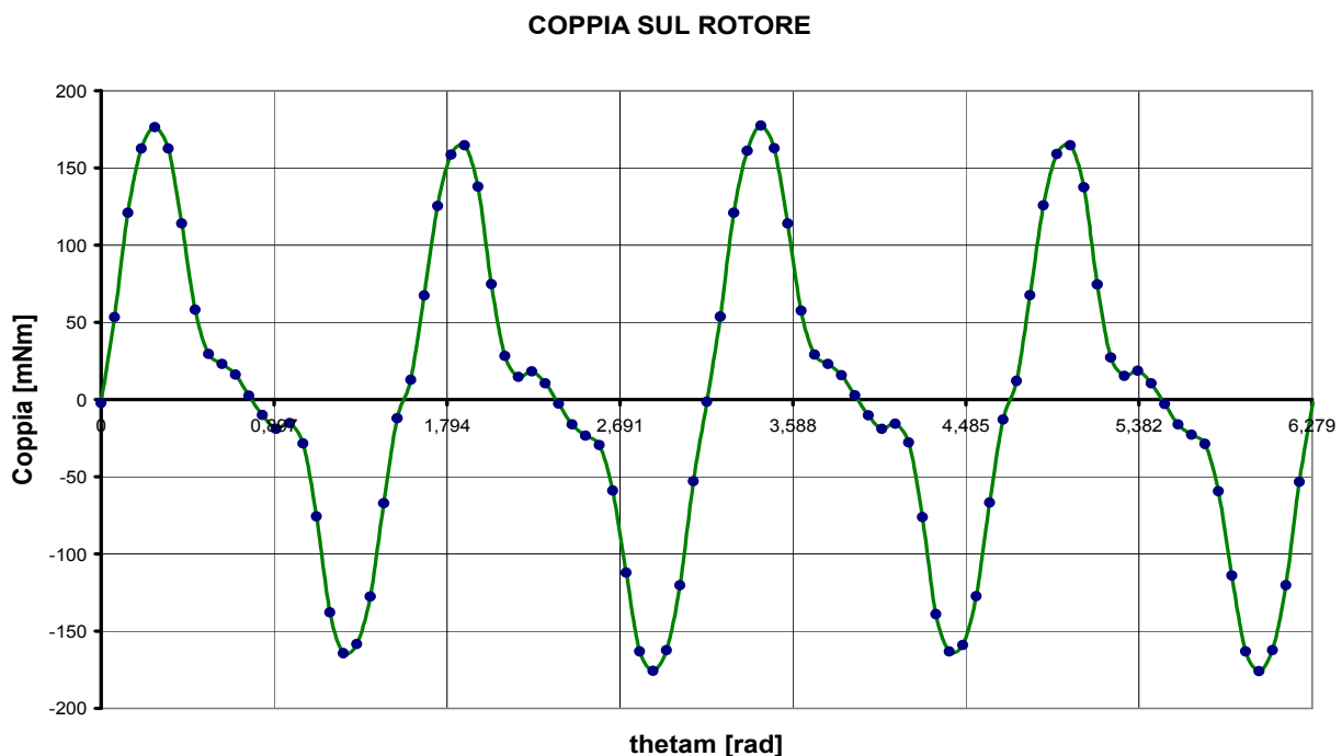
Fig. 7.45: Coppia a vuoto ottenuta mediante programma di simulazione FEMM
