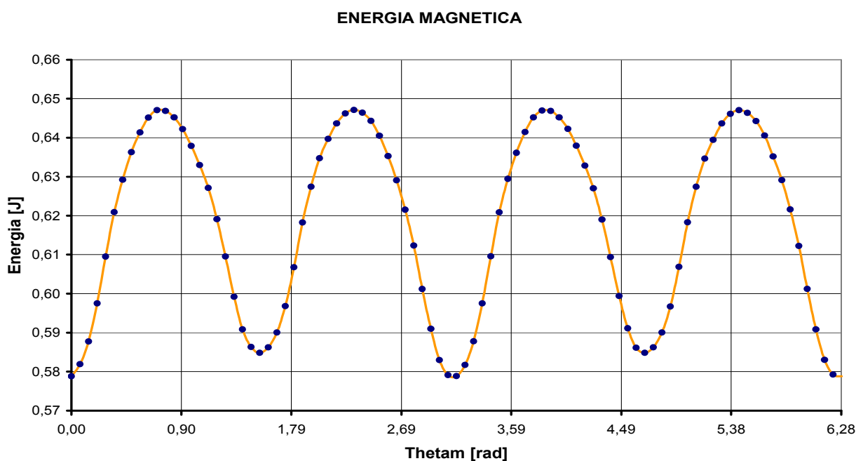
Fig. 7.29: Energia magnetica in funzione di \theta_m in regime continuo per \omega_m = 170 [rad/s]
