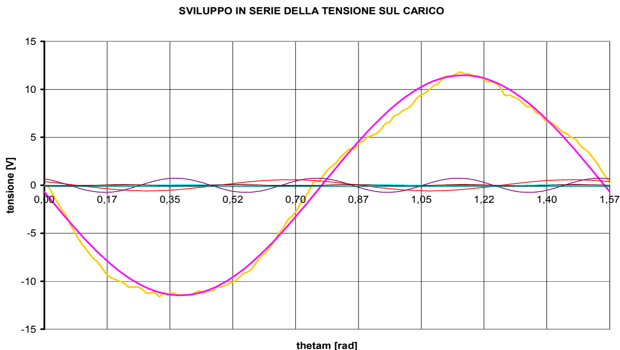
Fig. 5.7: Sviluppo in serie di Fourier della tensione applicata al carico
