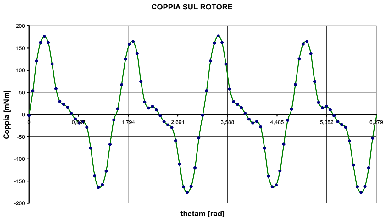
Fig. 7.50: Coppia a vuoto ottenuta mediante programma di simulazione FEMM
