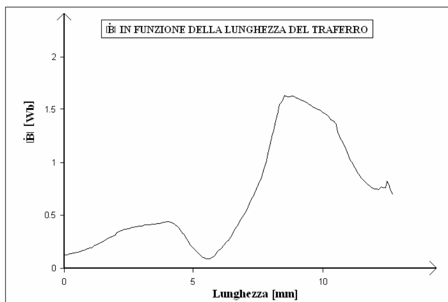
Fig. 2.50: |\dot{B}| in funzione della lunghezza del traferro a carico (modello 2)
