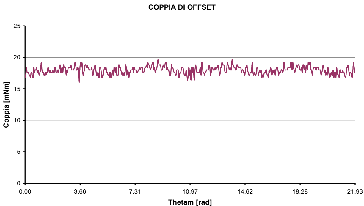
Fig. 7.43: Coppia di offset a vuoto misurata con torsionmetro meccanico per \omega_m = 10.74 [rad/s]
