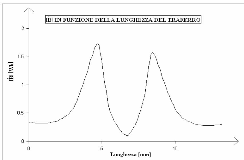
Fig. 2.76: |\dot{B}| al traferro in regime sinusoidale (modello 3)
