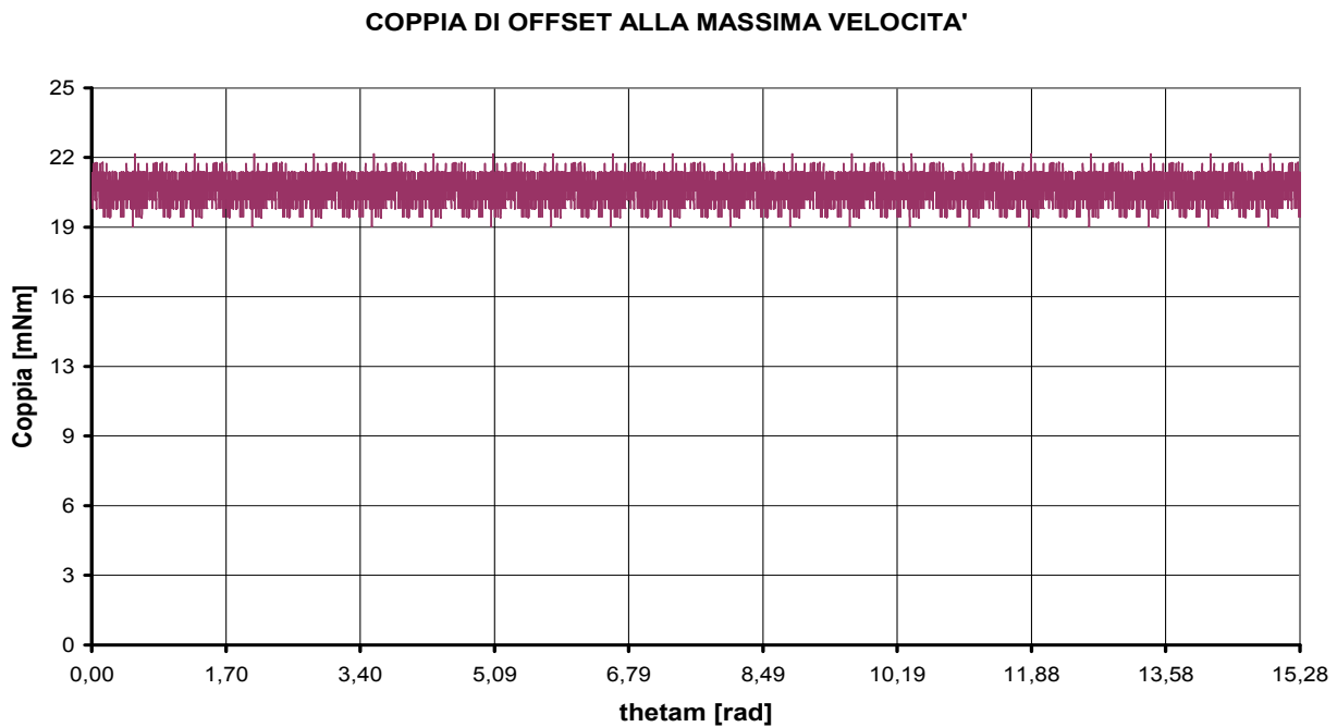
Fig. 5.19: Coppia di offset misurata con torsionometro meccanico per \omega_m = 154.12 [rad/s]
