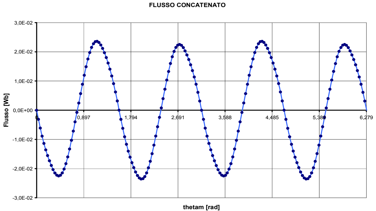
Fig. 2.68: Flusso concatenato in funzione di \theta_m (modello definitivo a vuoto)
