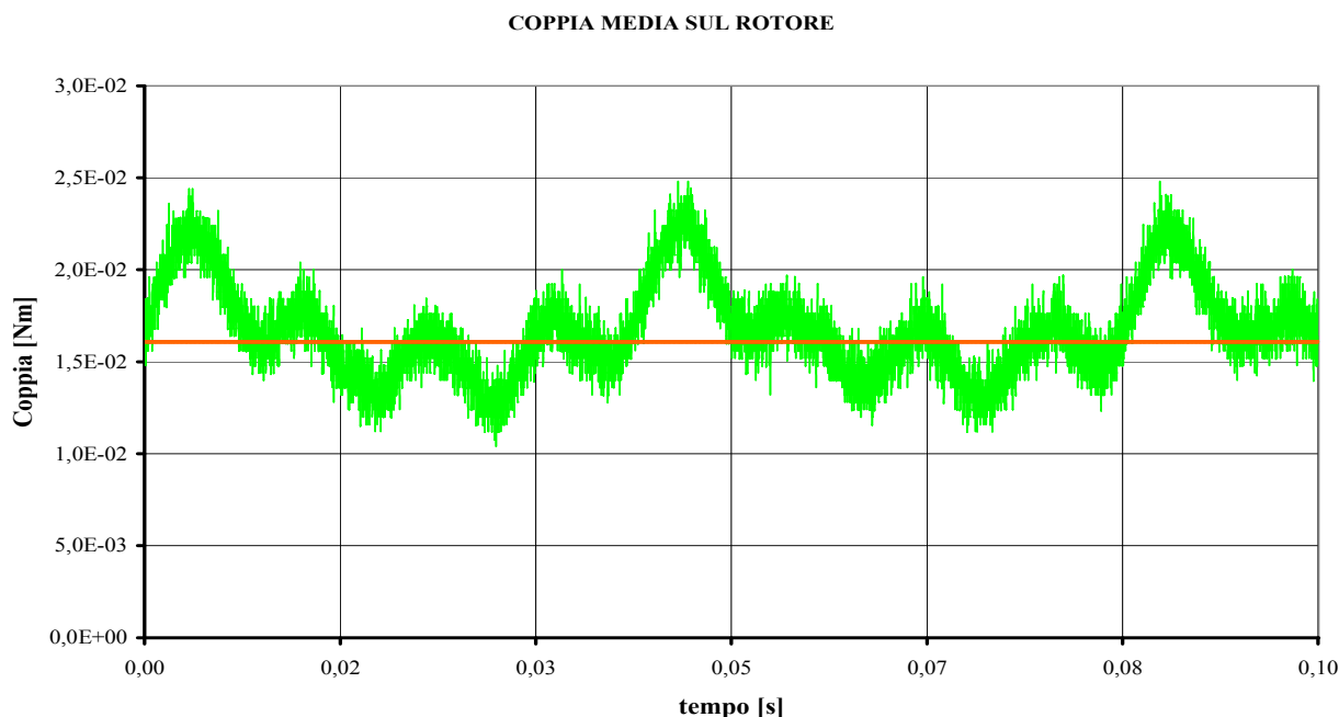
Fig. 6.12: Coppia media stimata a regime sinusoidale per \omega_m = 143.31 [rad/s] ed R = 5[\Omega]
