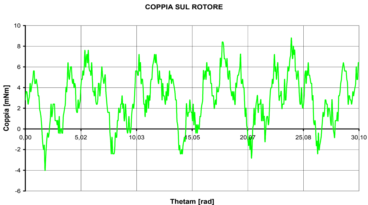
Fig. 7.62: Coppia al netto dell' offset misurata in regime continuo per \omega_m = 170 [rad/s]
