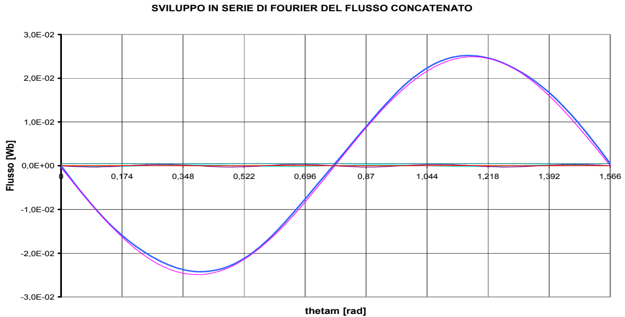
Fig. 7.14: Contenuto armonico del flusso \Phi_c(\theta_m) (funzionamento a vuoto)
