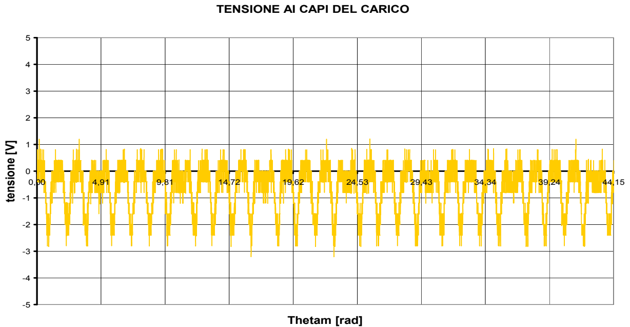
Fig. 5.12: Tensione generata a vuoto per \Omega_m = 10.74 [rad/s]
