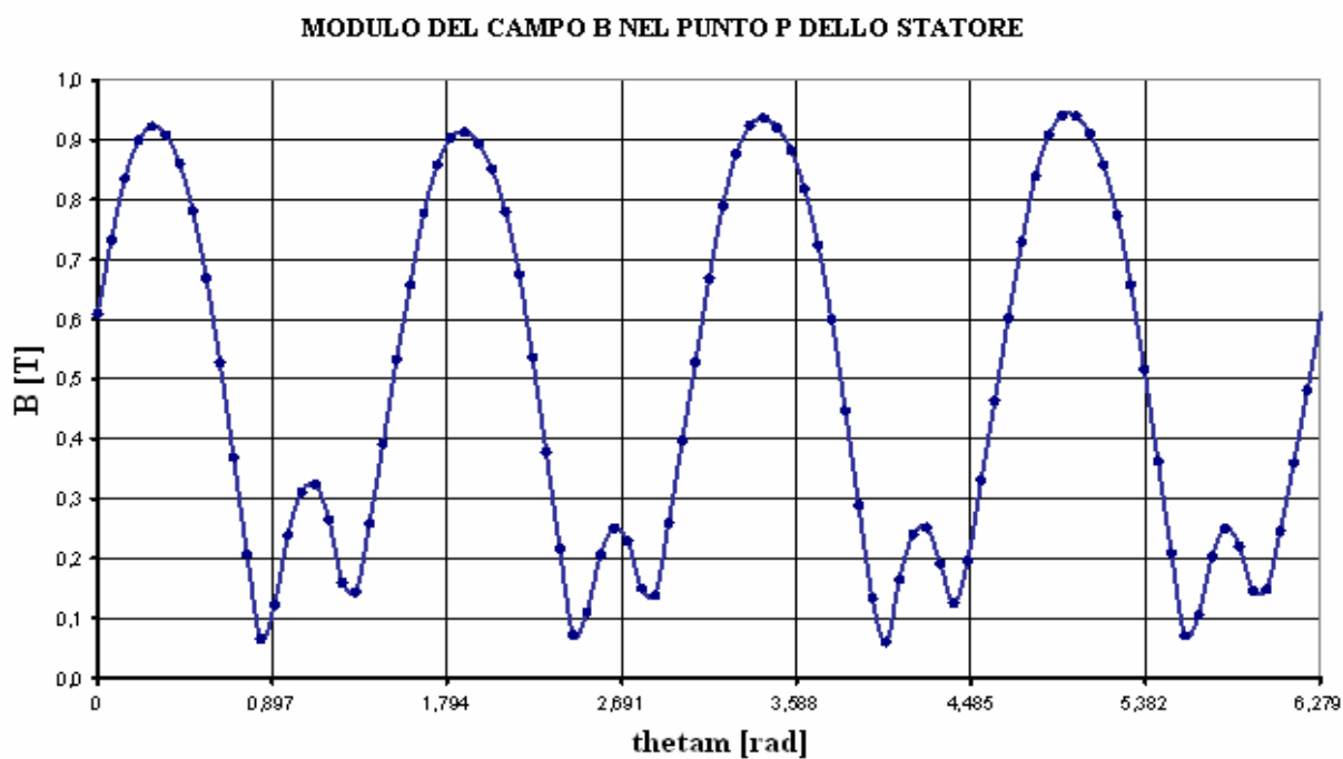
Fig. 6.5: Analisi del campo d' induzione magnetica \dot{B} nel punto P
