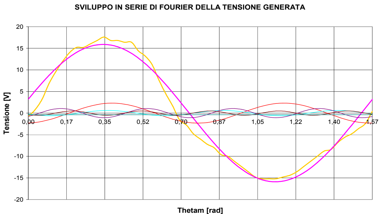
Fig. 7.37: Sviluppo in serie di Fourier della tensione a vuoto per \omega_m = 170 [rad/s]
