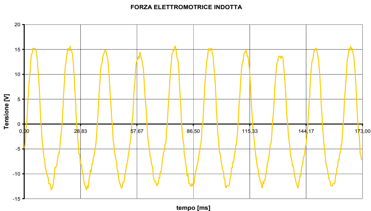
Fig. 7.38: Tensione applicata al carico resistivo in regime sinusoidale per \omega_m = 170 [rad/s]
