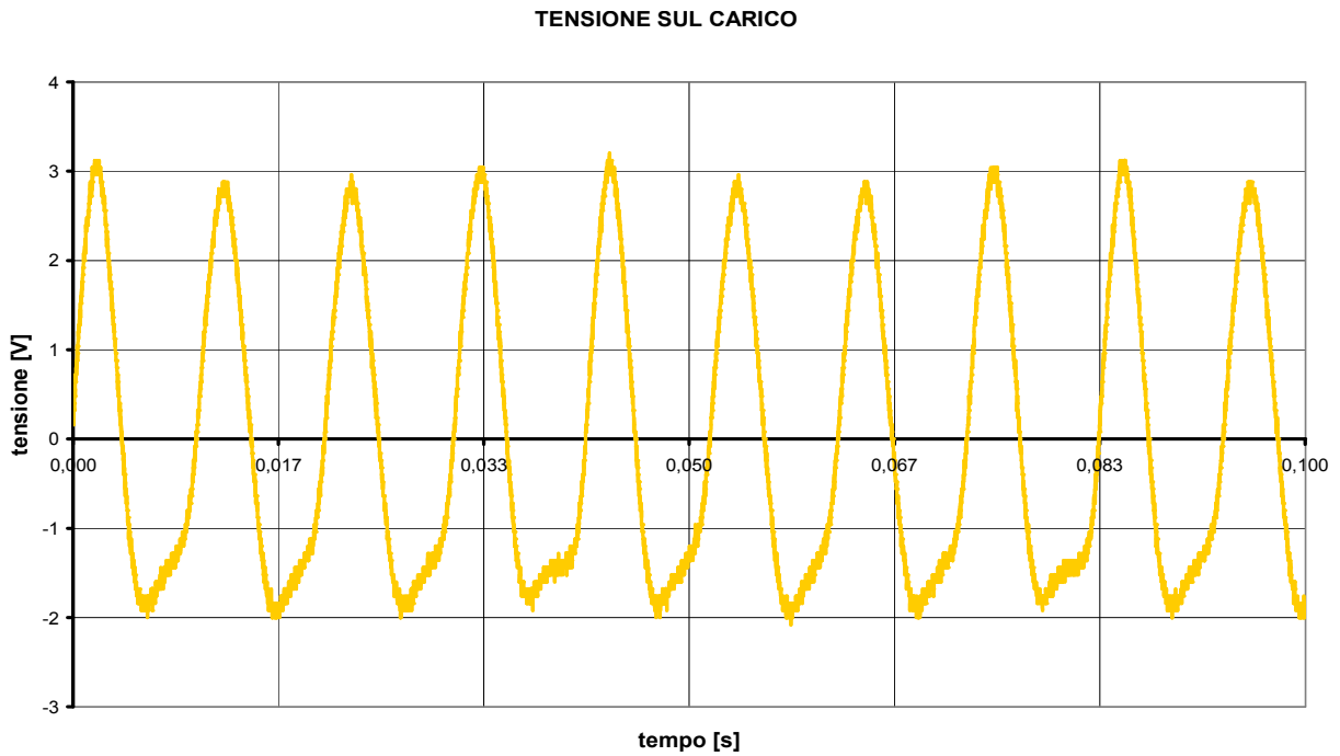
Fig. 6.13: Tensione ai capi del carico resistivo per \omega_m = 143.31[rad/s]
