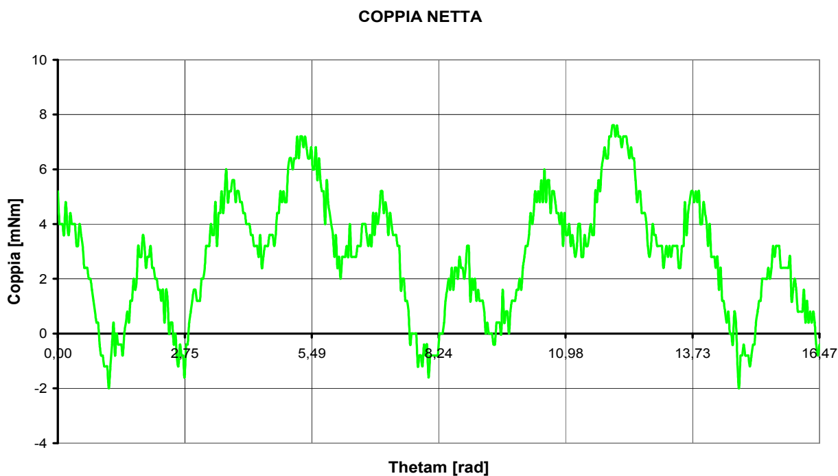
Fig. 7.49: Coppia netta a vuoto misurata con torsionometro meccanico per \omega_m = 170 [rad/s]
