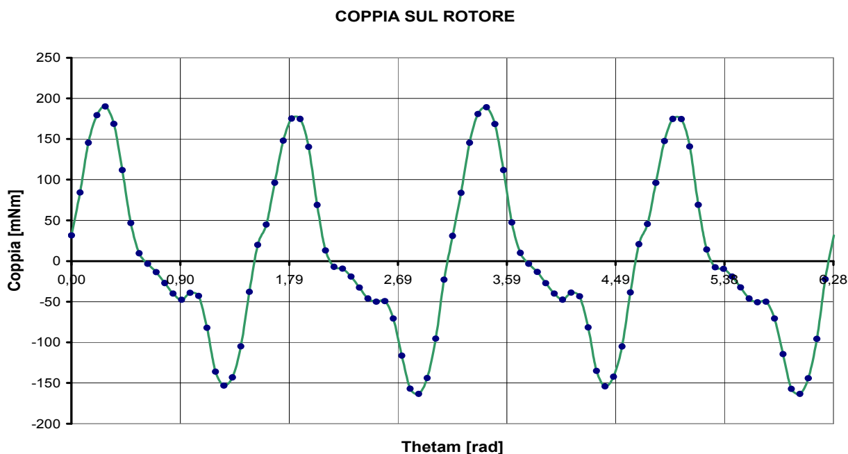
Fig. 7.28: Coppia sul rotore in funzione di \theta_m in regime continuo per \omega_m = 170 [rad/s]
