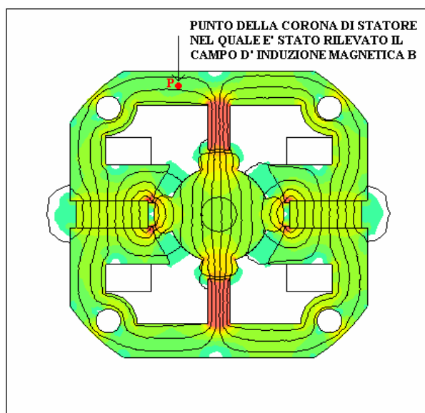
Fig. 6.4: Punto dello statore scelto per l'analisi del campo \dot{B}
