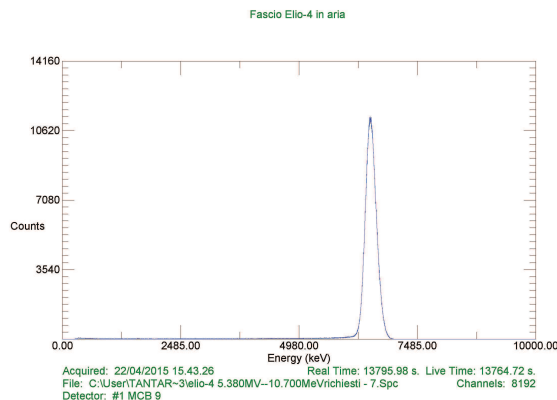
Figura 4.2: Spettro d'energia del fascio di particelle \alpha (in aria) da 6,5MeV. A seguito dell'attraversamento del foglio di mylar alla base della capsula di Petri, l'energia delle particelle \alpha incidenti sulle cellule è di 5,8MeV. Il LET corrispondente a quest'ultimo fascio di particelle \alpha è di 77 \frac{keV}{\mu m} .
