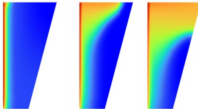
Figura 14 - Contour di temperatura geometria alternativa ciclo: 1, 3, 5
