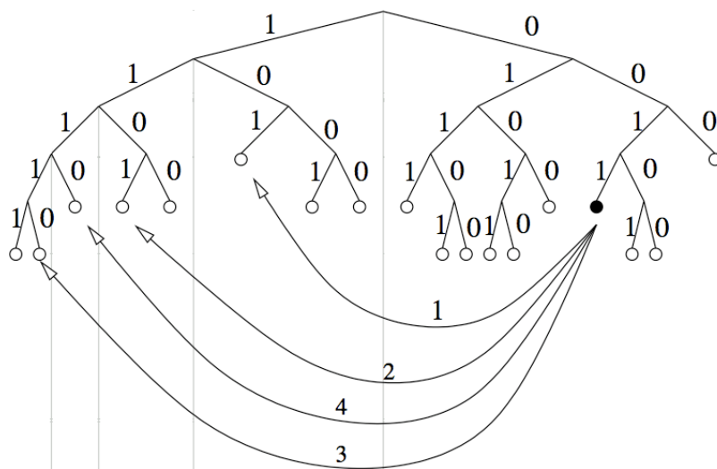
Figura 2.2: Passi dell'algoritmo in Kademia dal nodo 0011... al nodo 1110... mediante successive query.
