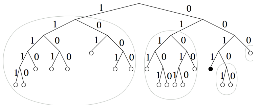
Figura 2.1: Albero binario di una rete Kademia. In nero è evidenziata la posizione di un nodo 0011... nell'albero. Cerchiati in grigio ci sono i sottolaberi in cui il nodo 0011... deve avere un contatto.
