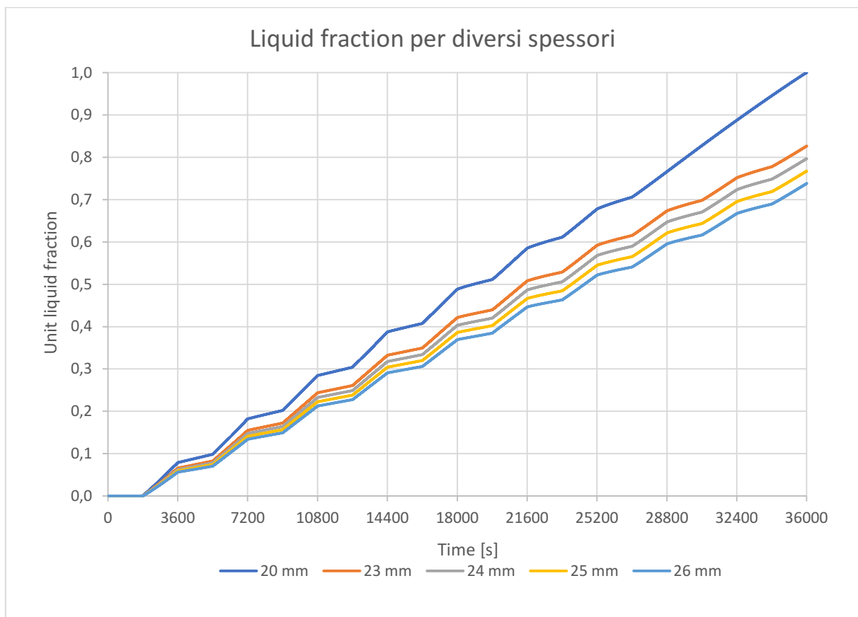
Fig.10 Grafico di comparazione del liquid fraction, a diversi spessori, durante i 10 cicli.
