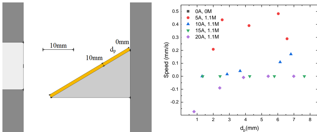
Figura 3.6- A sinistra: configurazione utilizzata per la misura. A destra: Velocità della goccia in funzione della posizione di deposito per diverse correnti immesse.
