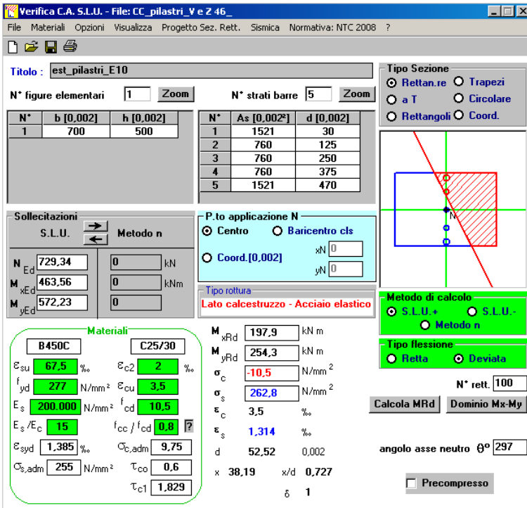
Figura 6.18. Inserimento parametri pil V46 Estratto VcaSlu del prof. Gelfi
