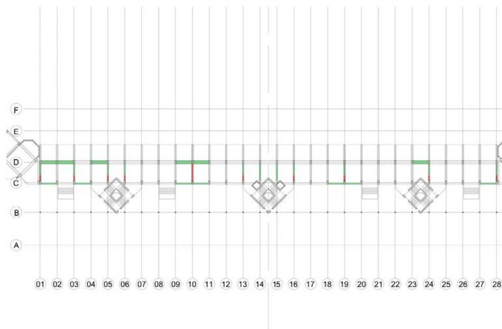
Figura 6.31. Analisi verifica pressoflessione Quota 9,45
