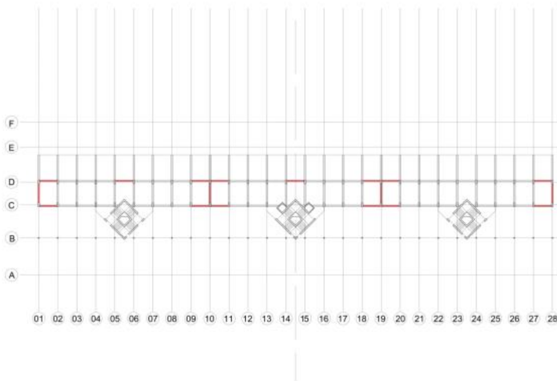
Figura 8.9. Intervento con setti strutturali in calcestruzzo armato Tribuna Est, quota 14,65
