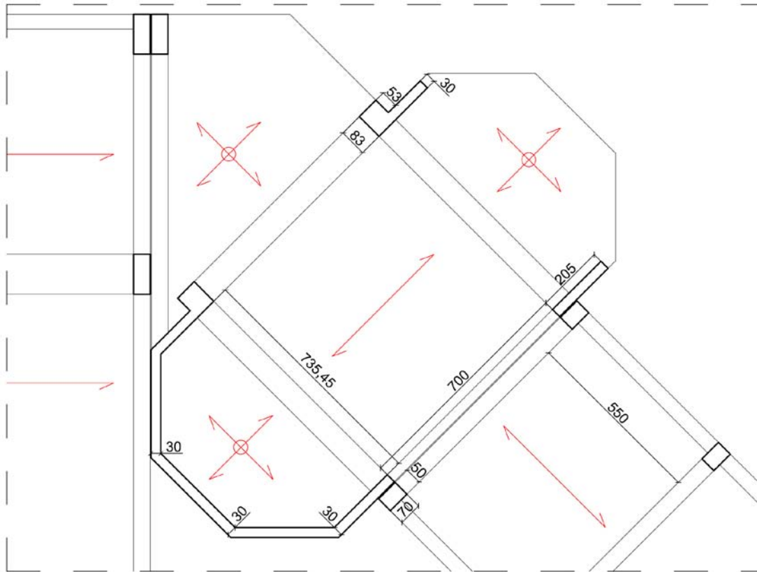
Figura 4.43. Dettaglio corpo di collegamento Corpo di collegamento Nord - Est
