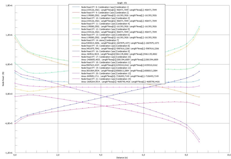
Figura 6.25. Grafico reazione vincolare R(y) Straus7
