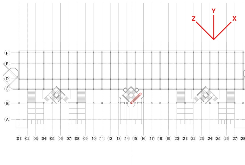
Figura 6.24. Localizzazione del setto analizzato Tribuna Est
