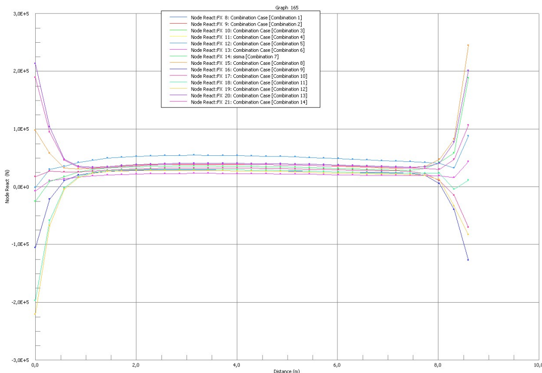
Figura 6.22. Grafico reazione vincolare R(x) Straus7
