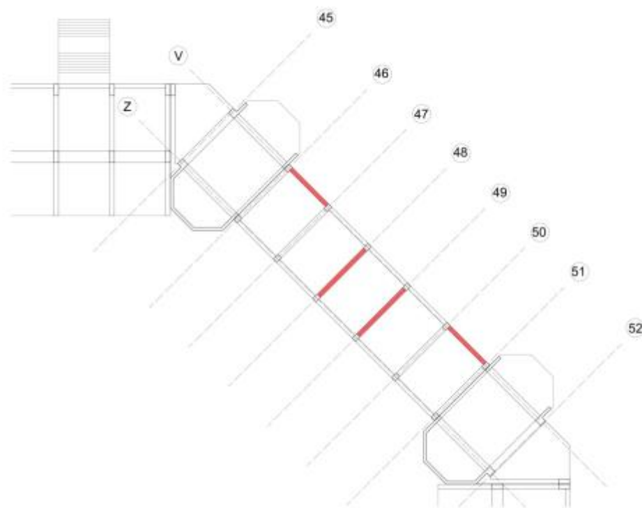
Figura 8.23. Intervento con setti strutturali in calcestruzzo armato Corpo di Collegamento, quota 9,45
