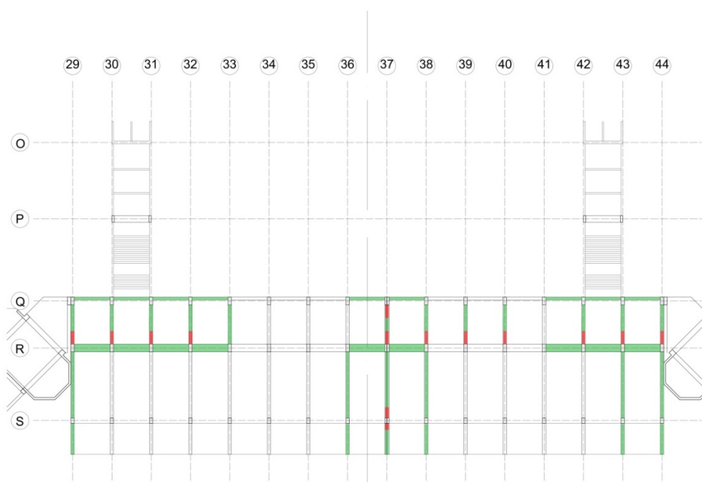
Figura 6.41. Risultati analisi taglio Quota 5,75
