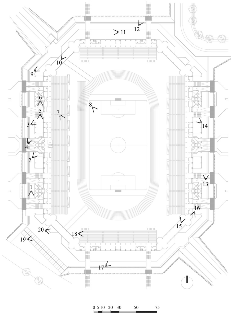
Figura 4.1. Inquadramento rilievo fotografico esterno Pianta quota 9,45
