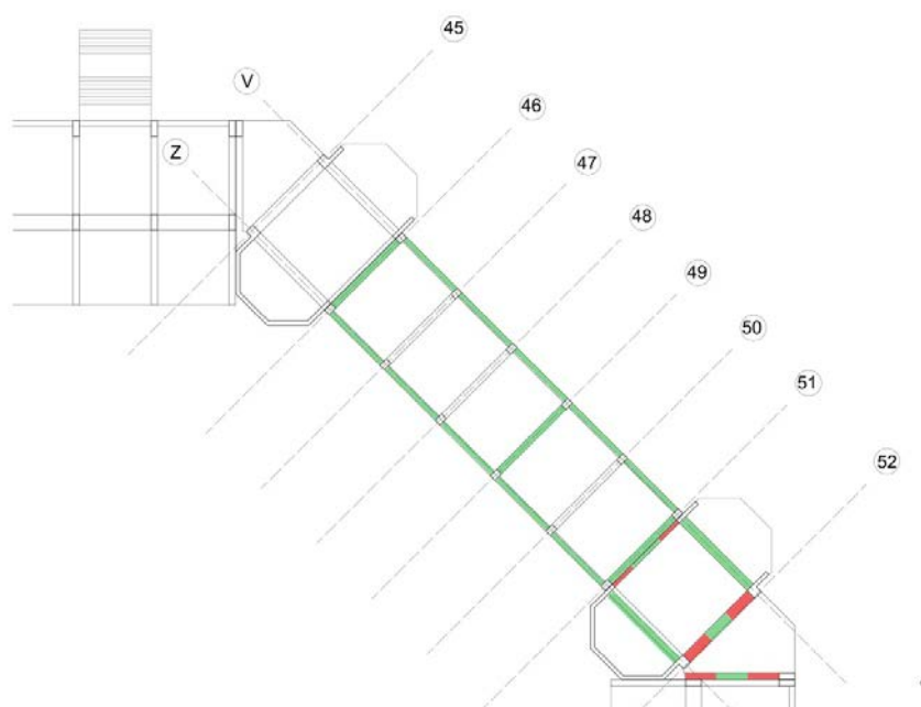
Figura 6.51. Analisi verifica taglio Quota 5,75
