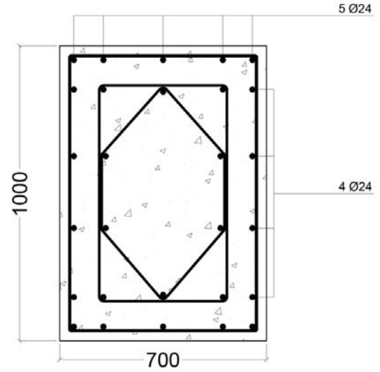
Figura 8.20. Dettagli costruttivi prima e dopo l'intervento proposto Tribuna Sud, fila S
