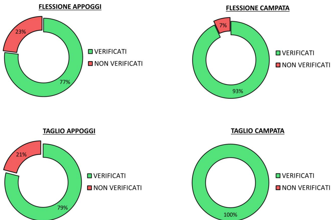
Figura 6.28. Riassunto delle verifiche
