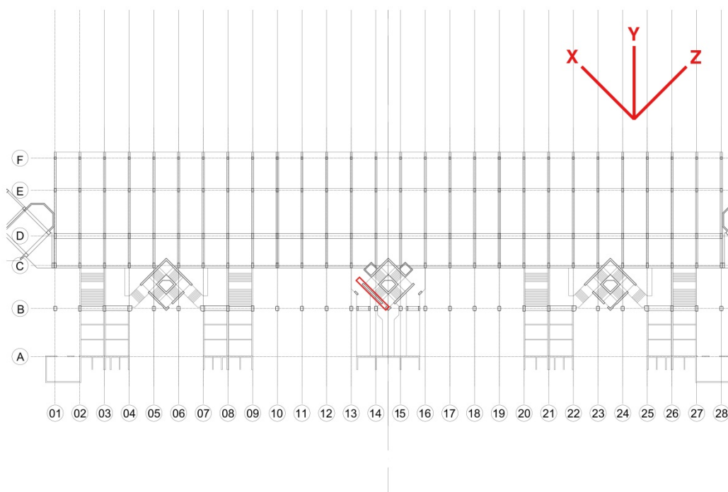
Figura 6.20. Localizzazione del setto analizzato Tribuna Est
