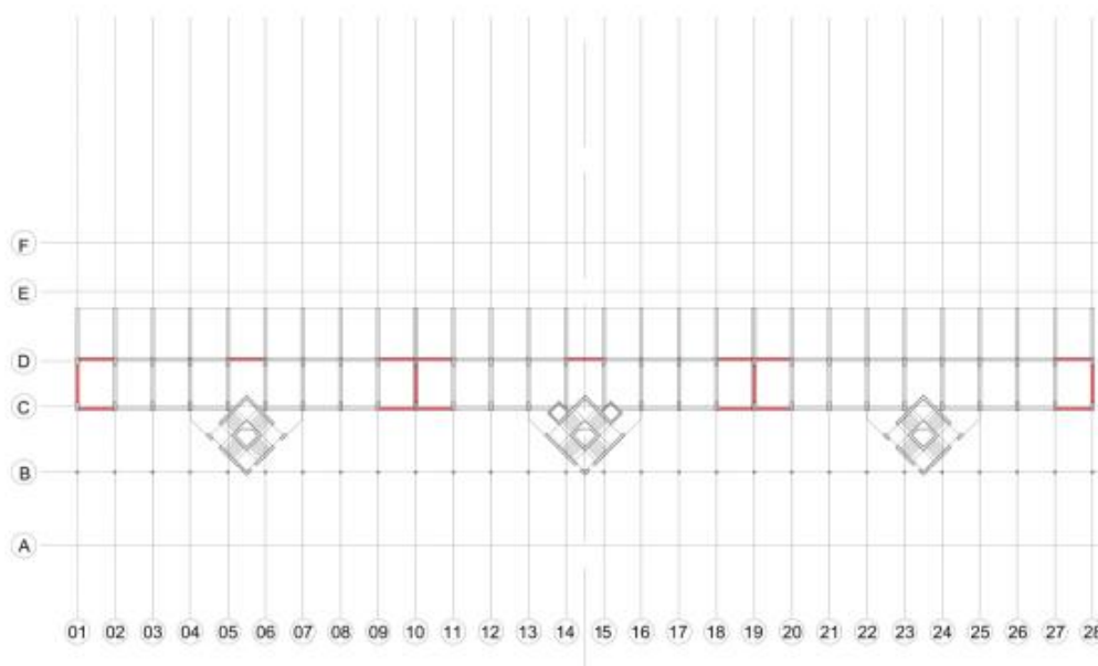
Figura 8.10. Intervento con setti strutturali in calcestruzzo armato Tribuna Est, quota 19,85
