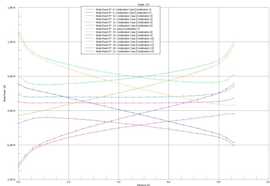
Figura 6.21. Grafico reazione vincolare R(y) Straus7
