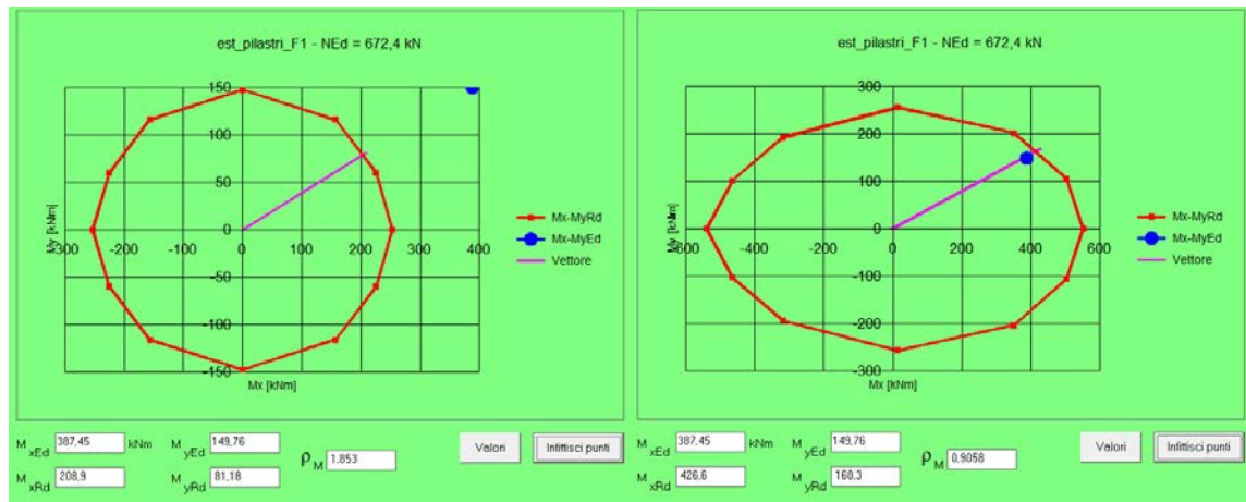
Figura 8.15. Dominio M-N prima e dopo l'intervento Tribuna Est, fila F
