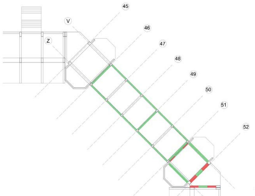
Figura 6.53. Analisi verifica taglio Quota 9,45
