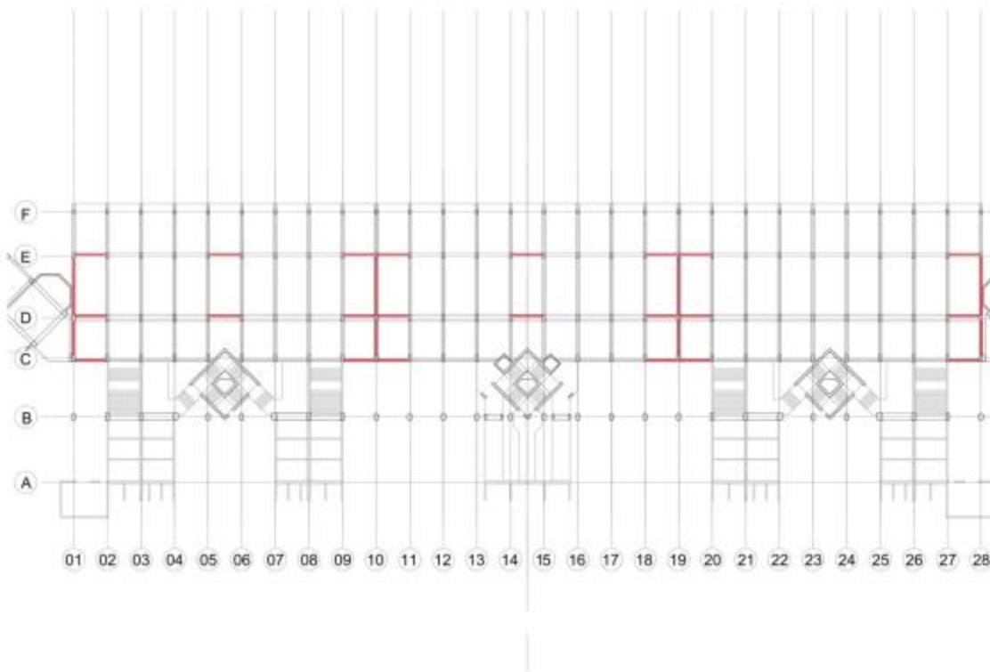
Figura 8.7. Intervento con setti strutturali in calcestruzzo armato Tribuna Est, quota 5,75
