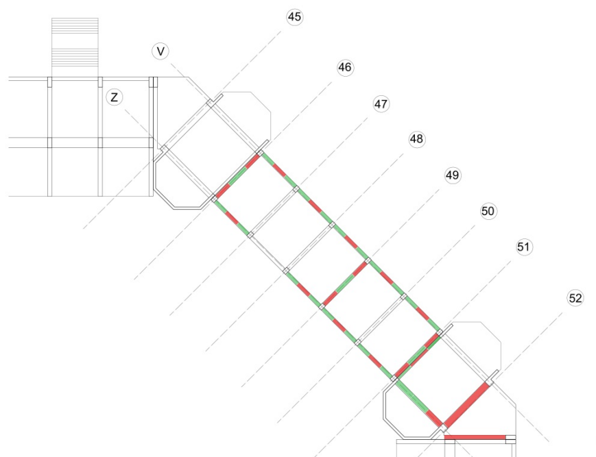
Figura 6.52. Analisi verifica pressoflessione Quota 9,45
