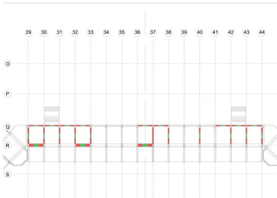
Figura 6.42. Analisi verifica pressoflessione Quota 9,45
