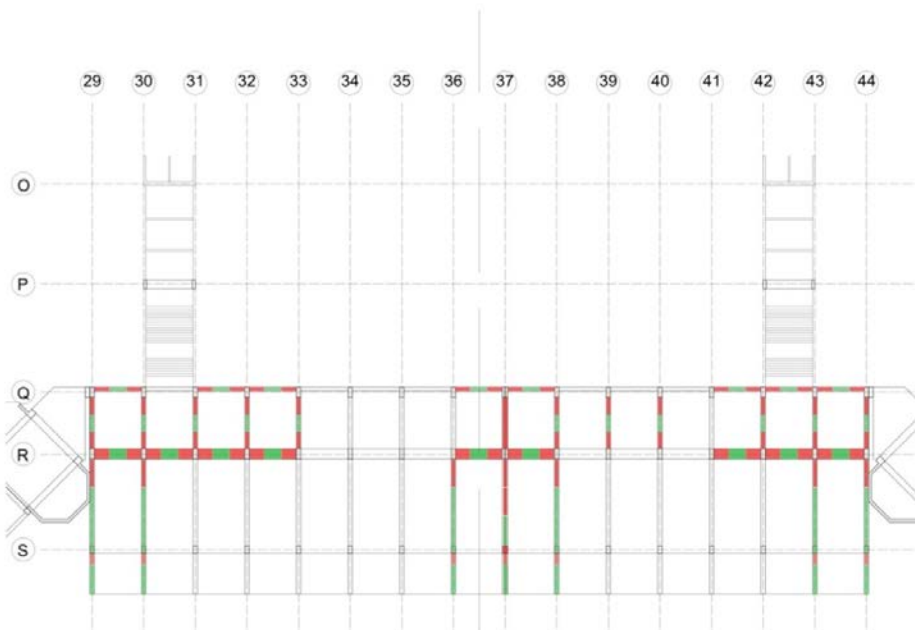
Figura 6.40. Analisi verifica pressoflessione Quota 5,75
