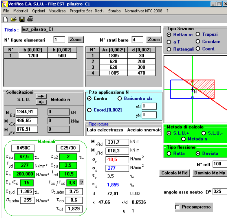
Figura 6.15. Inserimento parametri pil Q29 Estratto VcaSlu del prof. Gelfi
