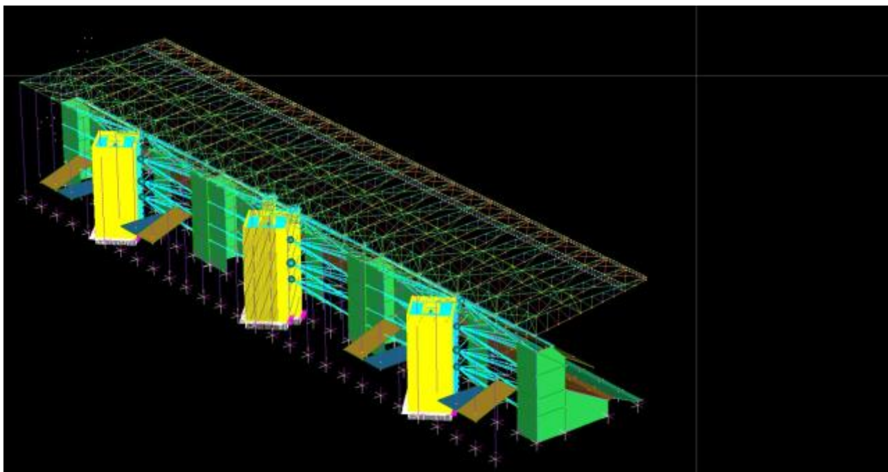
Figura 8.11. Modello Straus7 dell'intervento Tribuna Est
