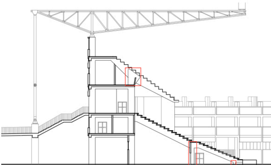
Figura 6.38. Dettaglio pilastri non verificati Sezione trasversale Tribuna Est
