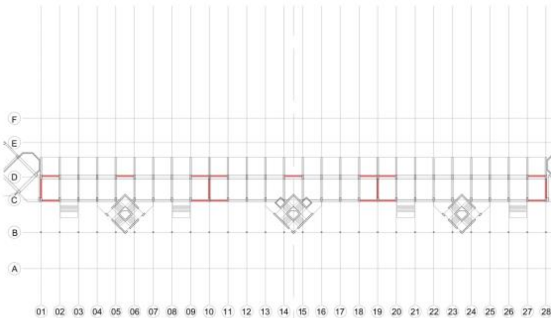
Figura 8.8. Intervento con setti strutturali in calcestruzzo armato Tribuna Est, quota 9,45
