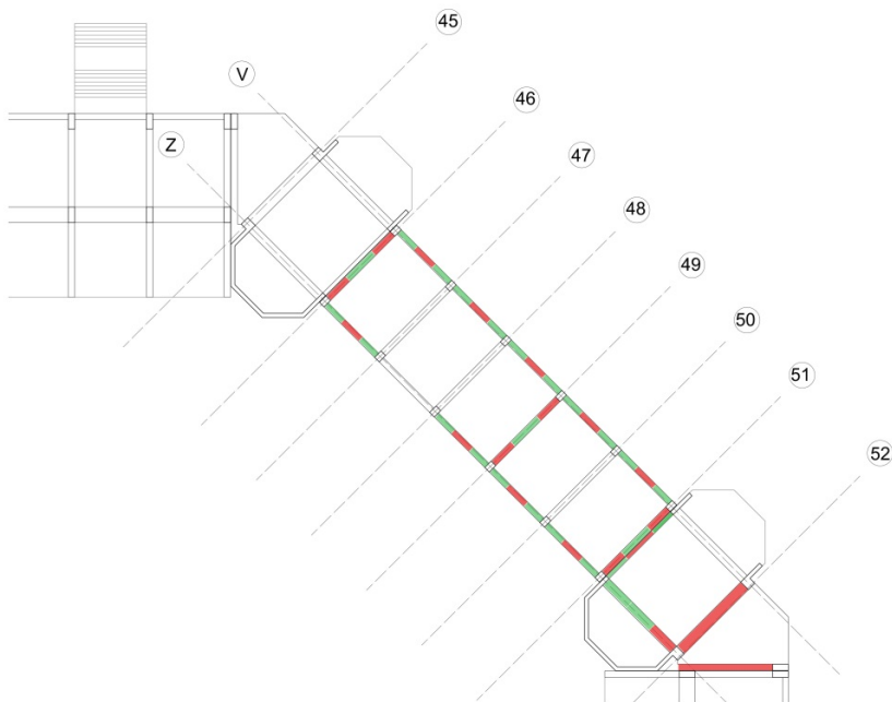
Figura 6.50. Analisi verifica pressoflessione Quota 5,75
