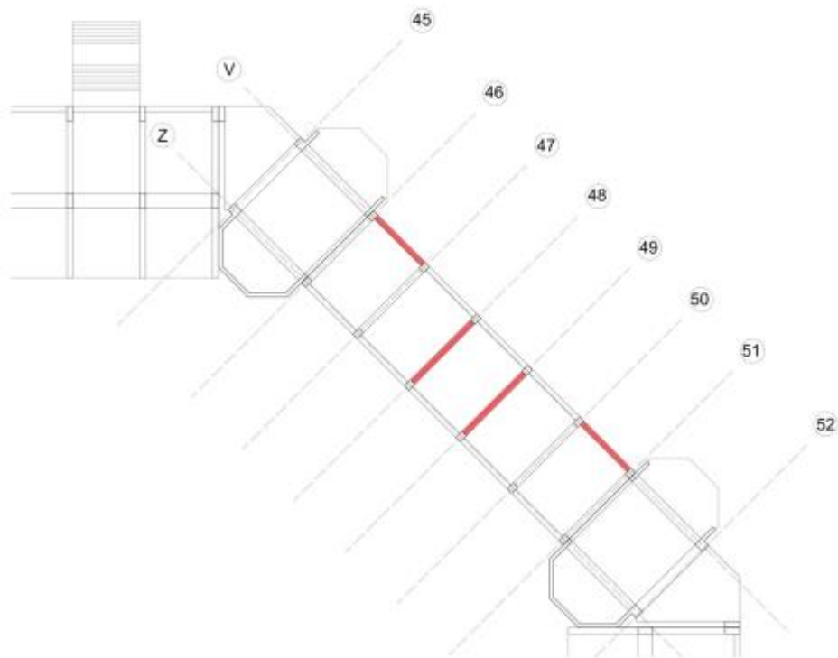
Figura 8.22. Intervento con setti strutturali in calcestruzzo armato Corpo di Collegamento, quota 5,75
