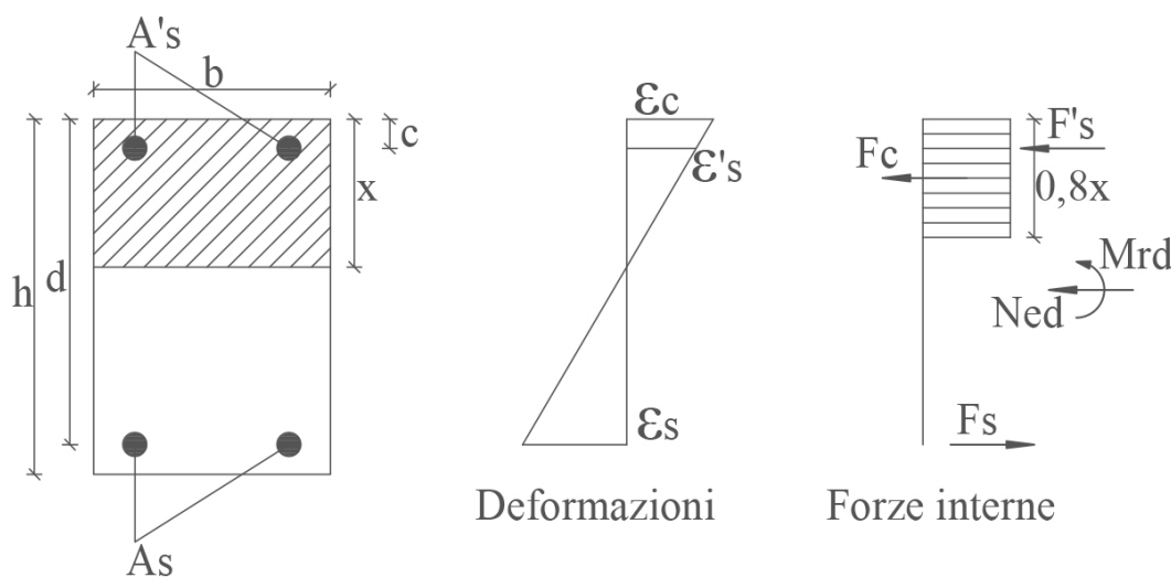
Figura 6.1. Grafico stress-block
