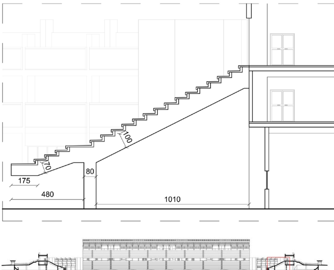
Figura 4.42. Dettaglio trave di sostegni gradinata Prospetto Tribuna Sud
