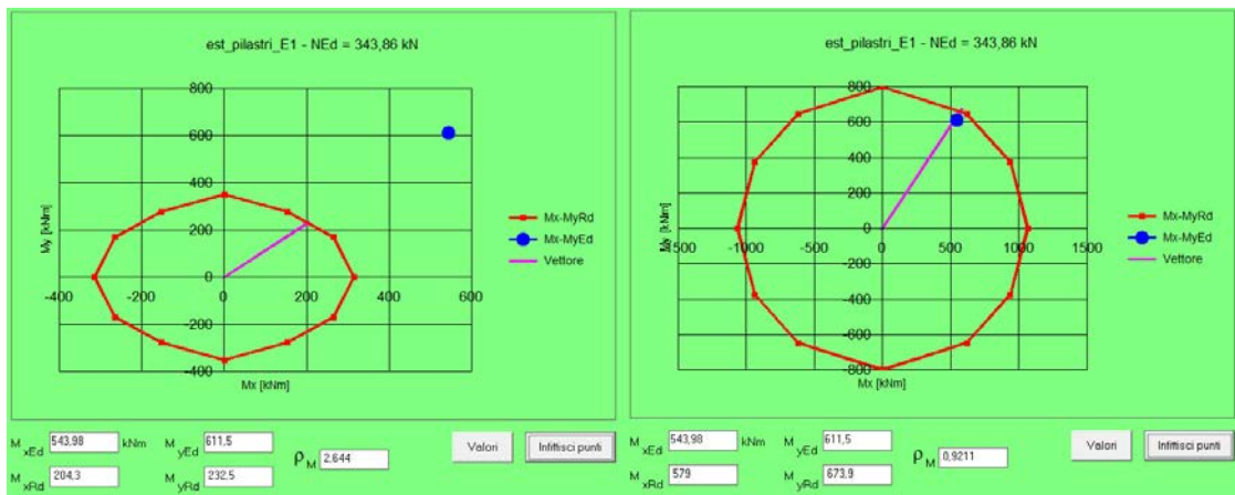
Figura 8.21. Dominio M-N prima e dopo l'intervento Tribuna Sud, fila S
