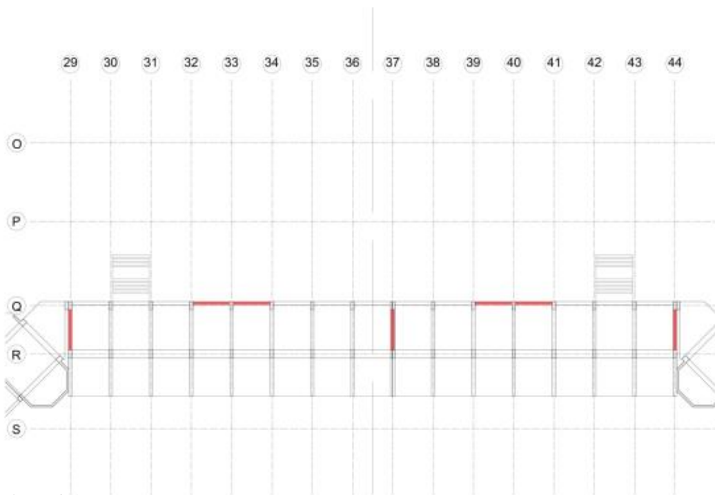
Figura 8.17. Intervento con setti strutturali in calcestruzzo armato Tribuna Sud, quota 9,45
