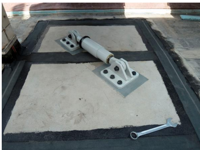
Figura 8.3. Esempio di dissipatore idraulico
