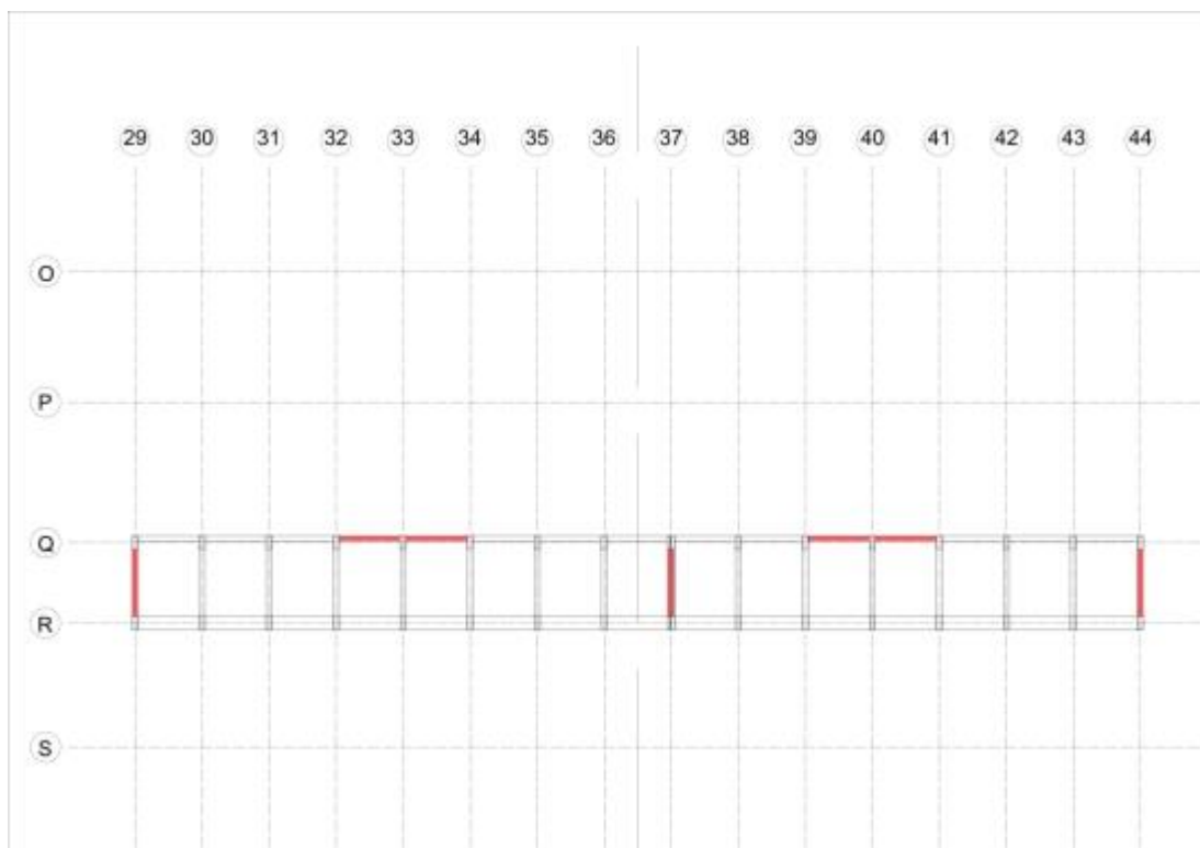
Figura 8.18. Intervento con setti strutturali in calcestruzzo armato Tribuna Sud
