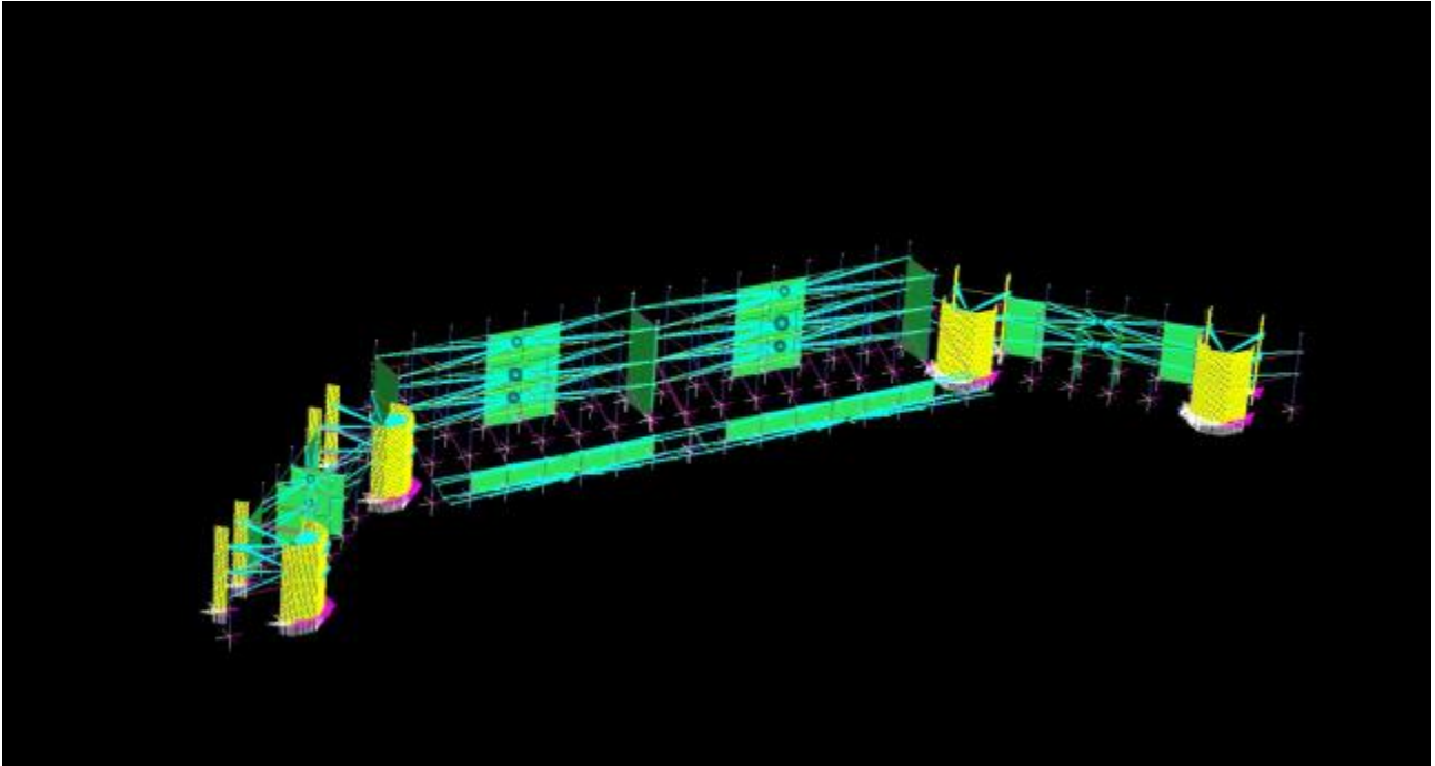
Figura 8.19. Modello Straus7 dell'intervento Tribuna Sud e corpi di collegamento
