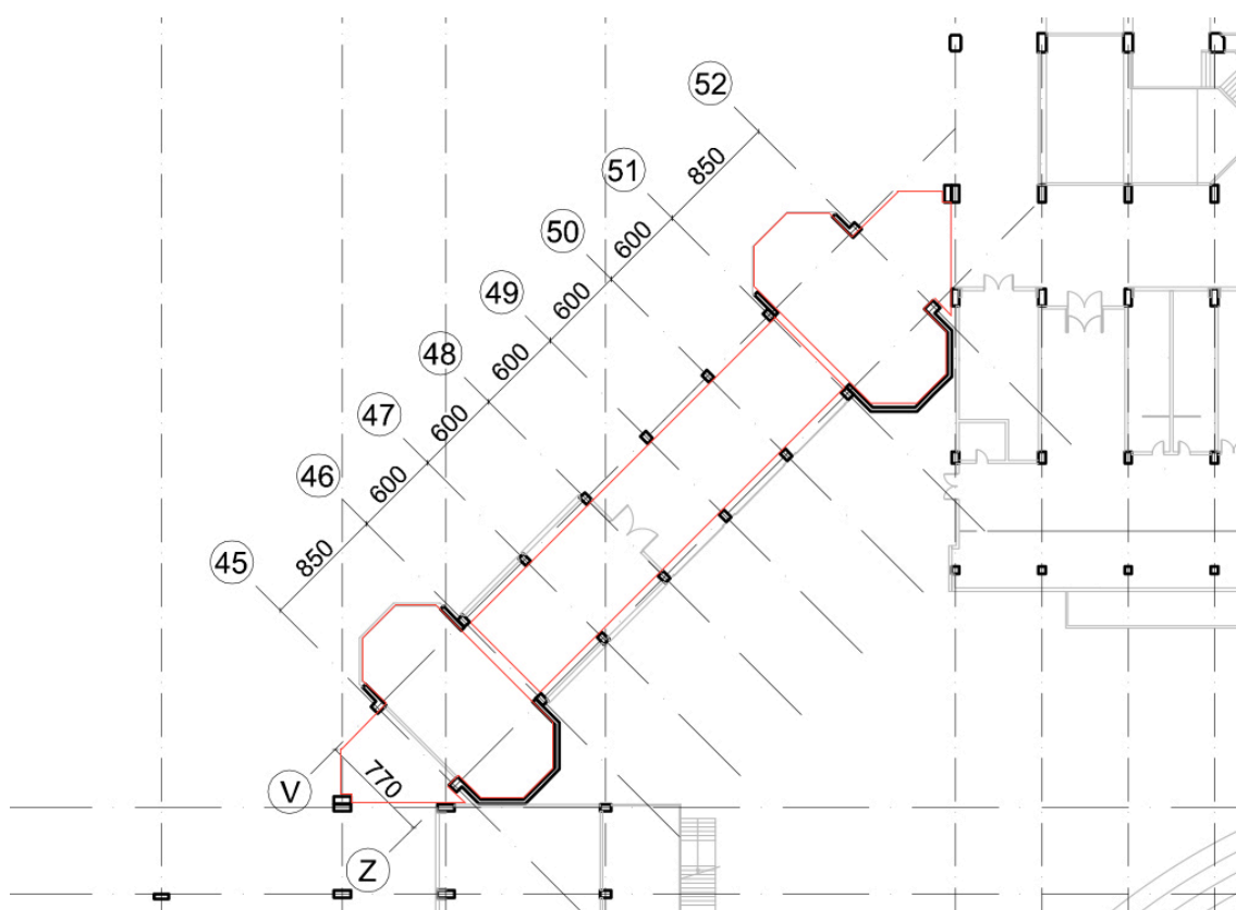
Figura 6.48. Suddivisione delle tre zone Dettaglio Corpo di collegamento
