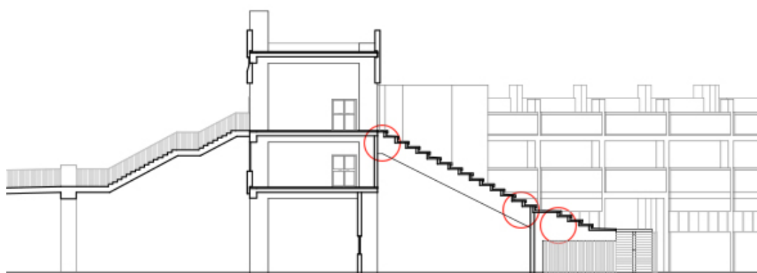
Figura 6.46. Dettaglio travi tribuna non verificate Sezione trasversale Tribuna Sud
