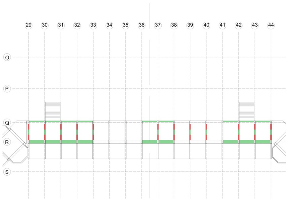
Figura 6.43. Analisi verifica pressoflessione Quota 9,45
