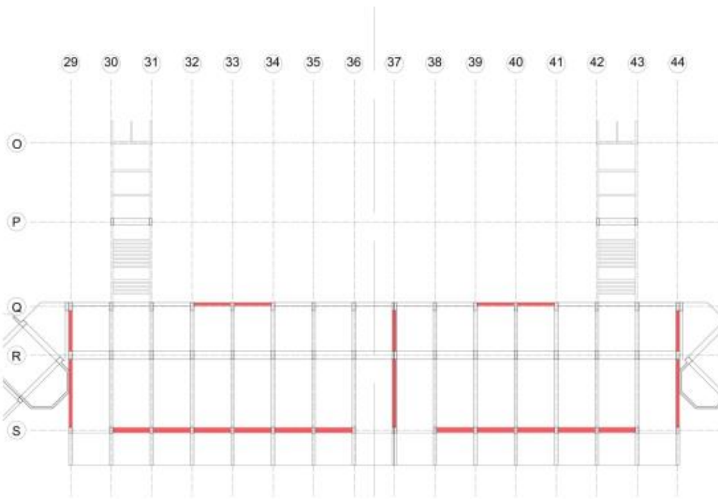
Figura 8.16. Intervento con setti strutturali in calcestruzzo armato Tribuna Sud, quota 5,75
