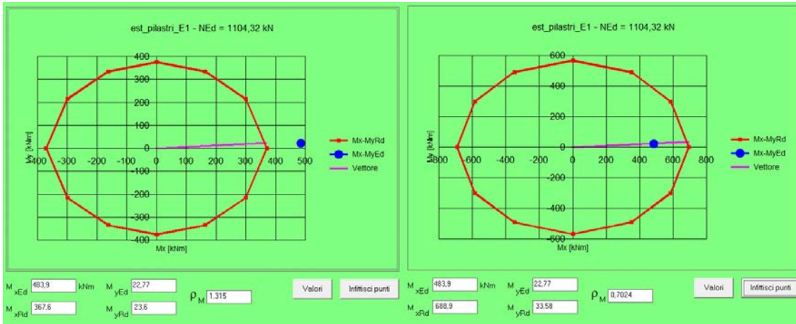
Figura 8.13. Dominio M-N prima e dopo l'intervento Tribuna Est, fila E
