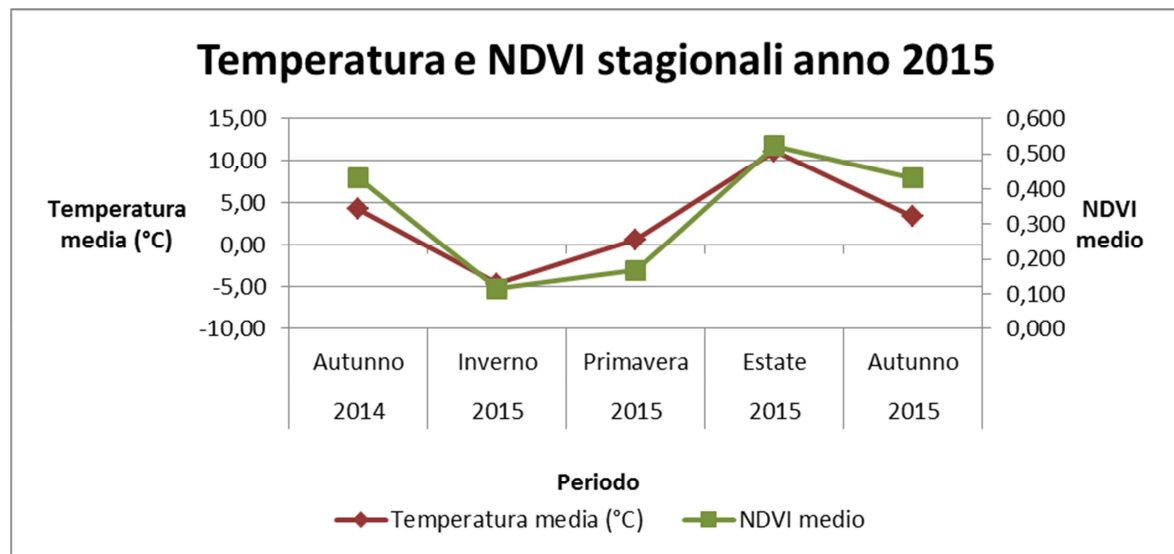
Grafico 4.7: Andamento stagionale della temperatura media e dell'NDVI medio nel 2015.
