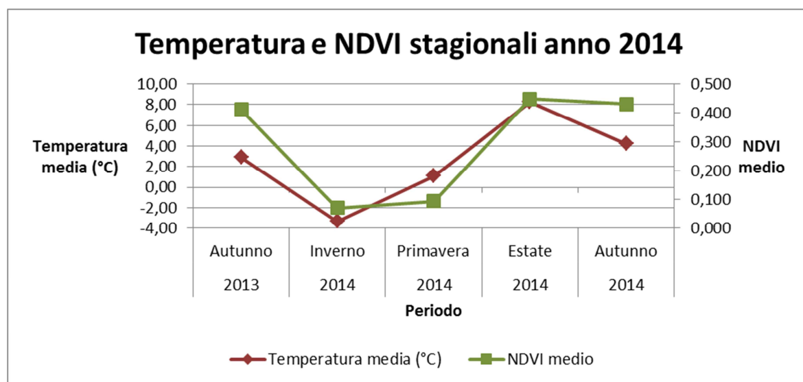
Grafico 4.5: Andamento stagionale della temperatura media e dell'NDVI medio nel 2014.
