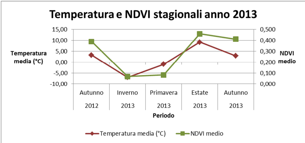
Grafico 4.3: Andamento stagionale della temperatura media e dell'NDVI medio nel 2013.
