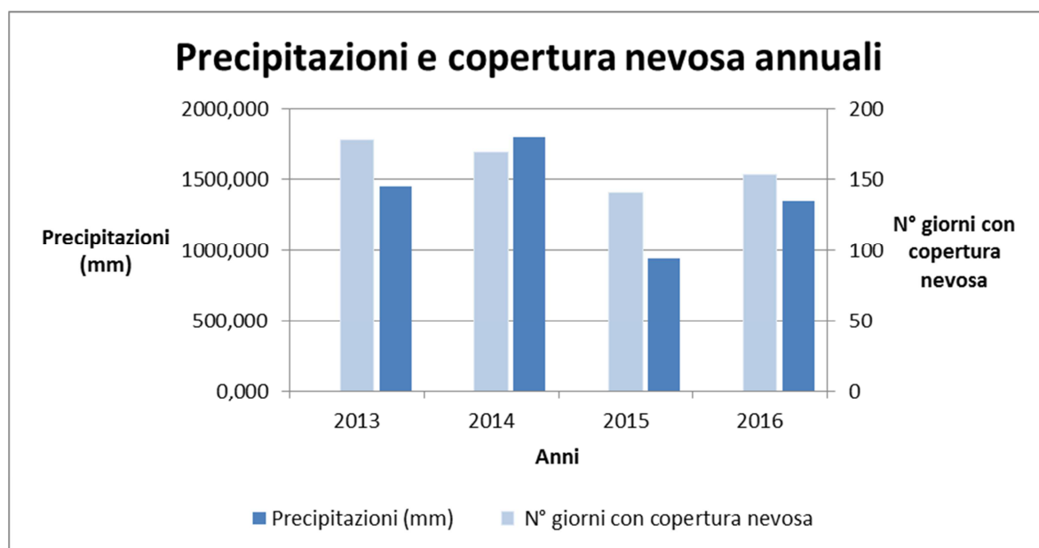
Grafico 4.2: Valori annuali di precipitazioni e n° di giorni con copertura nevosa.
