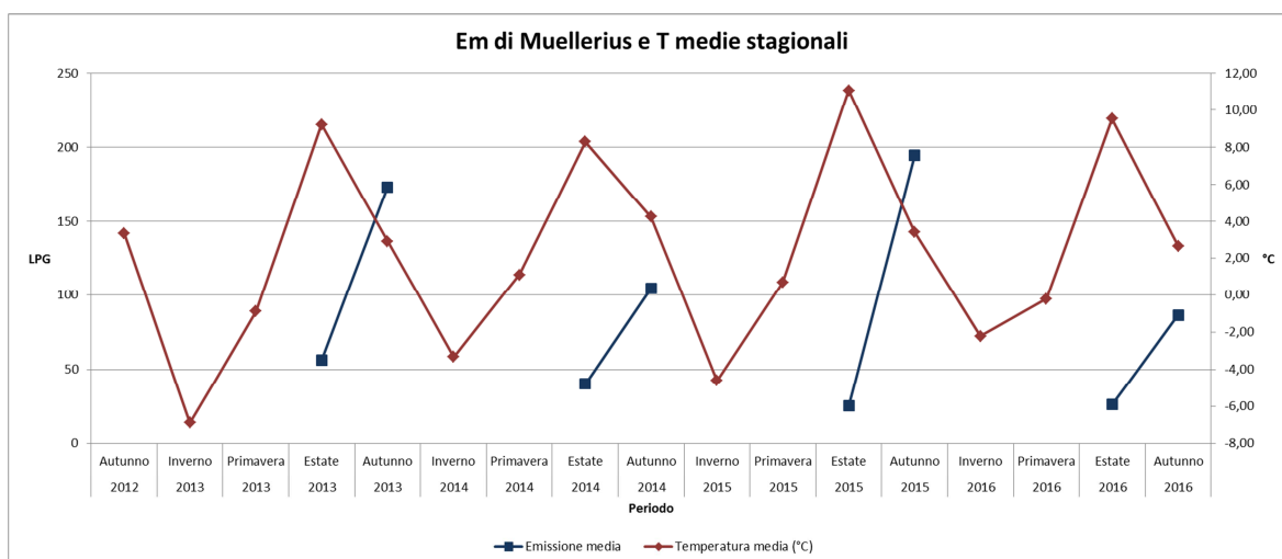
Grafico 4.16: T medie stagionali in relazione con l'Em stagionale nel corso degli anni.
