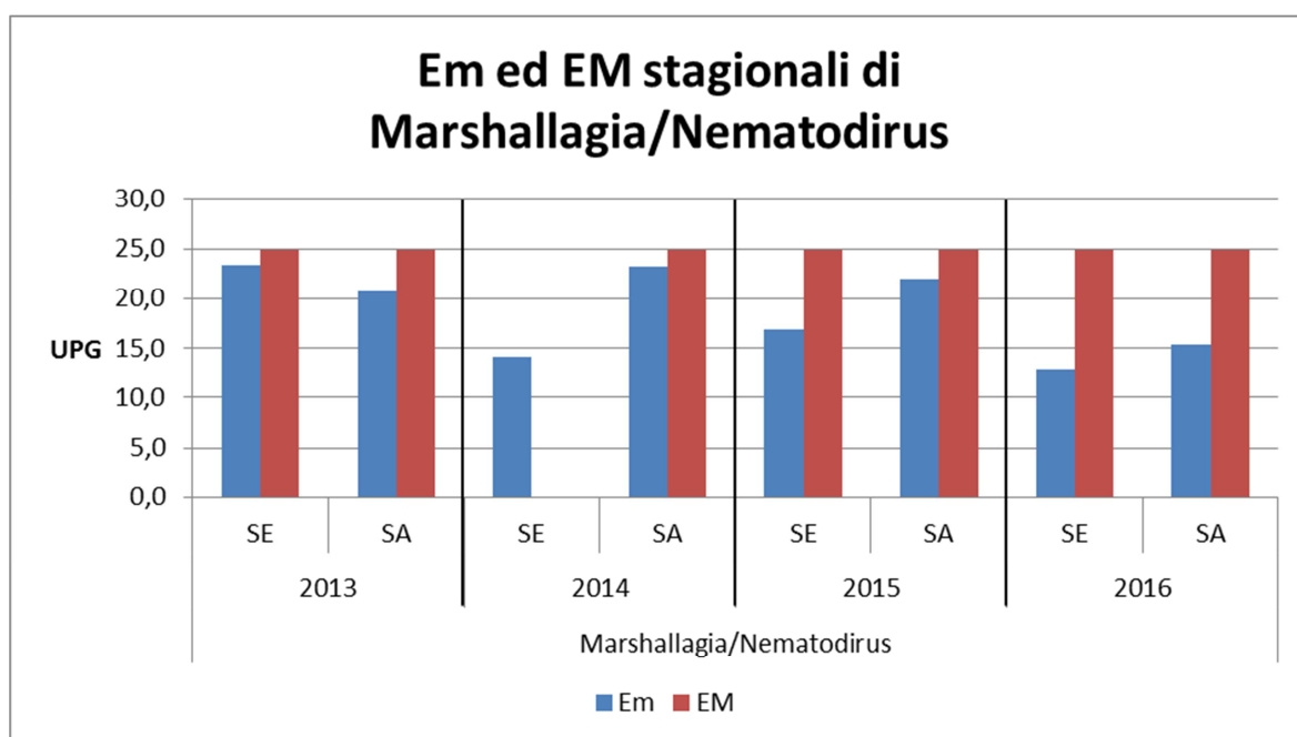
Grafico 4.13: Confronto tra l'Em e l'EM stagionali di Marshallagia/Nematodirus negli anni di studio
