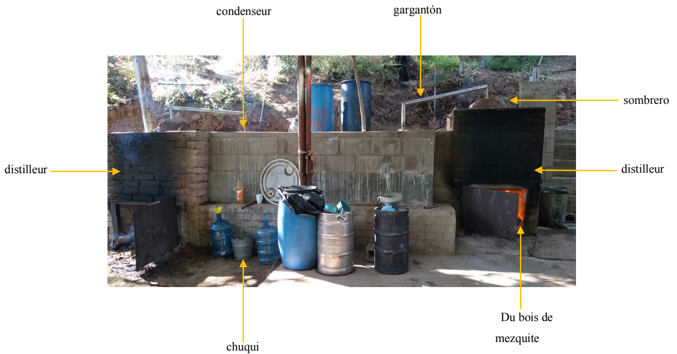
Figure 22. Système distillateur-condenseur
