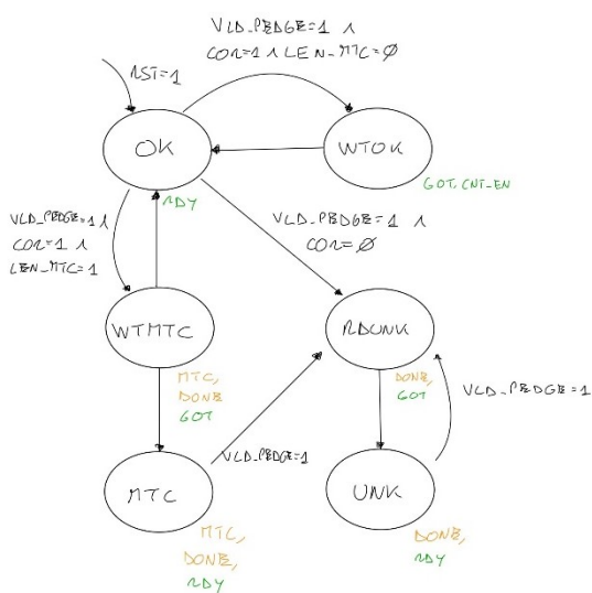
FIGURA 4-9 - DIAGRAMMA DI STATO DELL'ENTITY STATIC_RECOGNIZER
