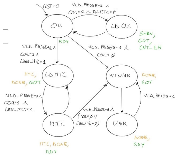
FIGURA 4-10 - DIAGRAMMA DI STATO DELL'ENTITY DYNAMIC_RECOGNIZER
