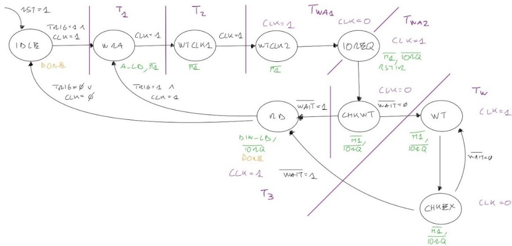
FIGURA 3-36 - DIGRAMMA DI STATO DELLA UFSM INTRQ
