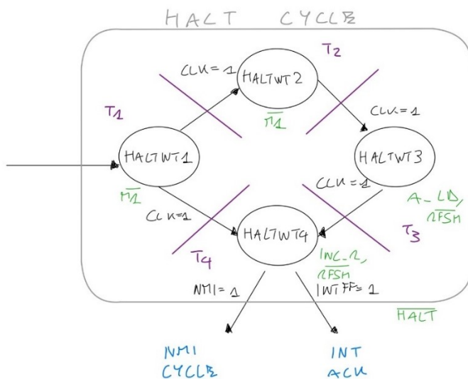
FIGURA 3-22 - DIAGRAMMI DI STATO DEL CICLO HALT CYCLE
