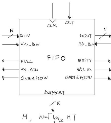
FIGURA 4-4 - SCHEMA DI UNA FIFO GENERICA
