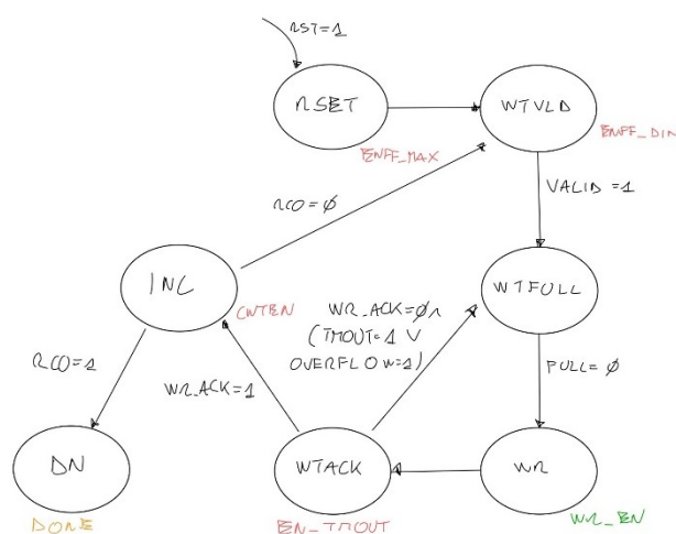
FIGURA 4-6 - DIAGRAMMA DI STATO DI CHAR_WRITER_FIFO
