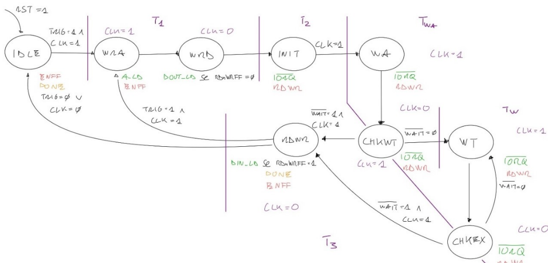
FIGURA 3-33 - DIGRAMMA DI STATO DELLA UFSM IORDWR
