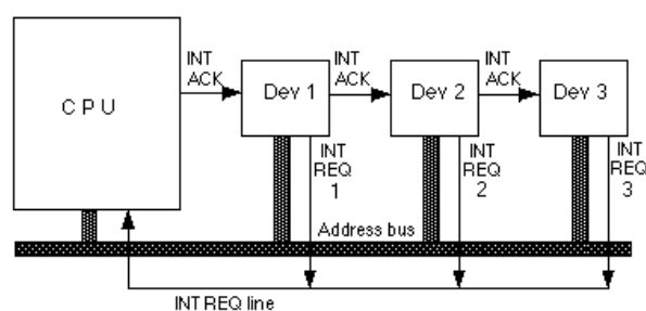
FIGURA 3-9 - ESEMPIO DI CONNESSIONE DAISY CHAIN. NELL'IMMAGINE L'ADDRESS BUS VIENE SOSTITUITO CON IL DATA BUS PER LO Z80.
