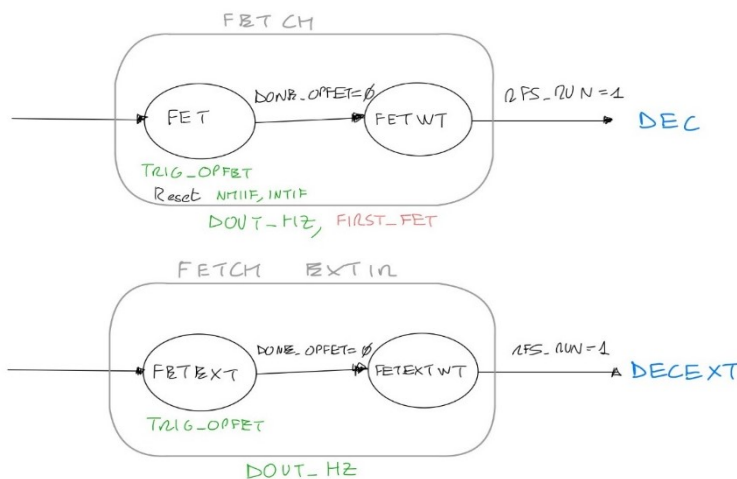
FIGURA 3-20 - DIAGRAMMI DI STATO DEI CICLI FETCH E FETCH EXTIR
