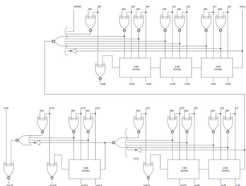
FIGURA 3-13 - CIRCUITO COMPLETO DELL'INC/DEC [27]
