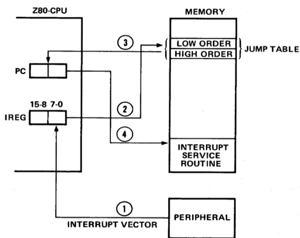
FIGURA 3-8 - SEQUENZA DI SERVIZIO DEGLI INTERRUPT VETTORIZZATI [24]
