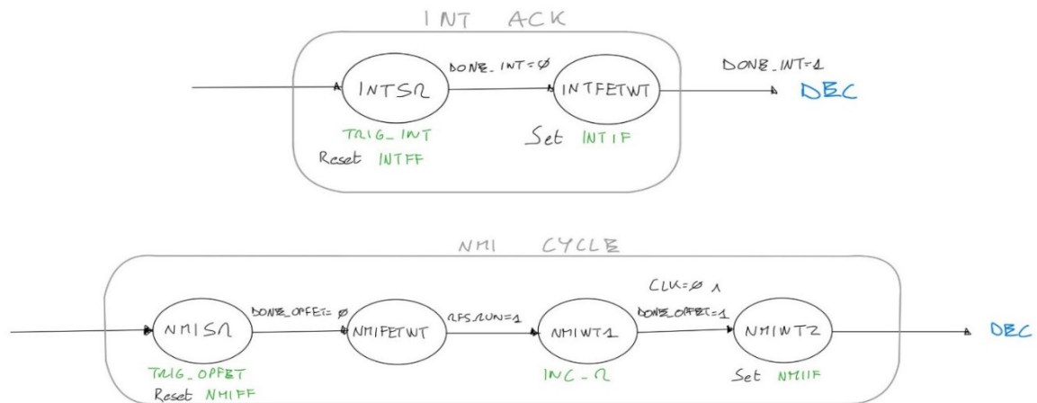
FIGURA 3-25 - DIAGRAMMI DI STATO DEI CICLI NMI CYCLE E INT ACK
