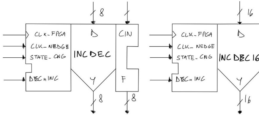
FIGURA 3-38 - SCHEMA DELL'INCDEC E INCDEC16
