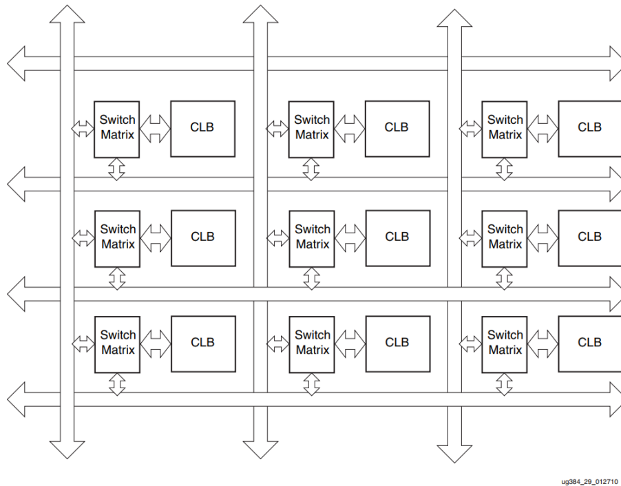
FIGURA 2-2 - SCHEMA DEI CLB E DEI CANALI D'INTERCONNESSIONE [9]
