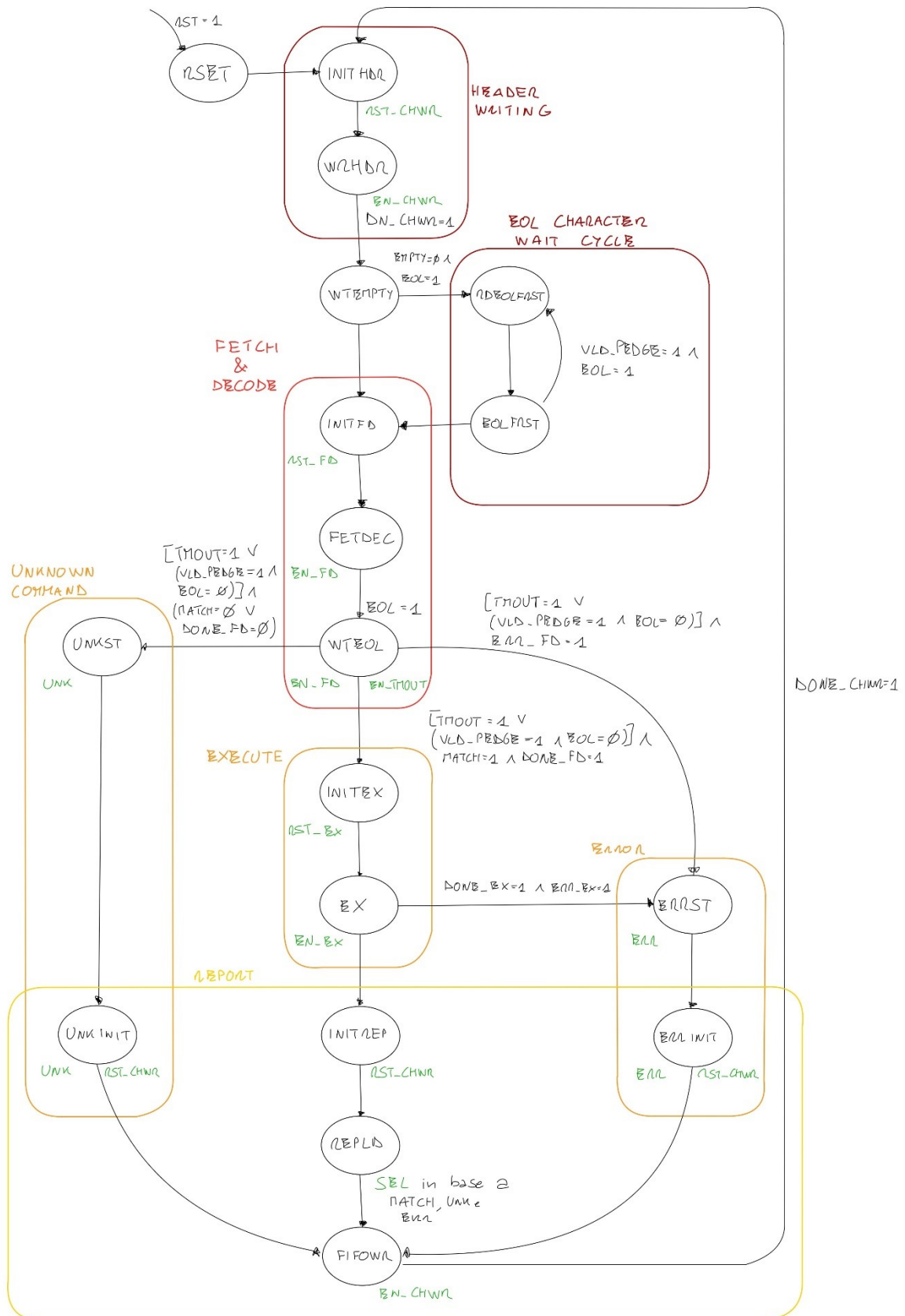
FIGURA 4-7 - DIAGRAMMA DI STATO DELLA FSM DI CMD_CTRL
