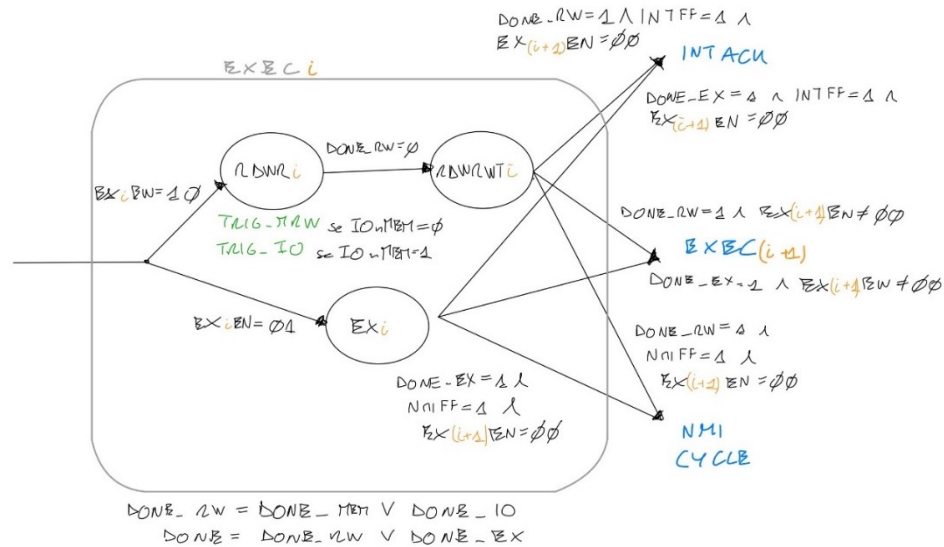
FIGURA 3-21 - DIAGRAMMI DI STATO DEI CICLI EXiEN, N INDICA L'INDICE DELLA FASE DI ESECUZIONE CORRISPONDENTE
