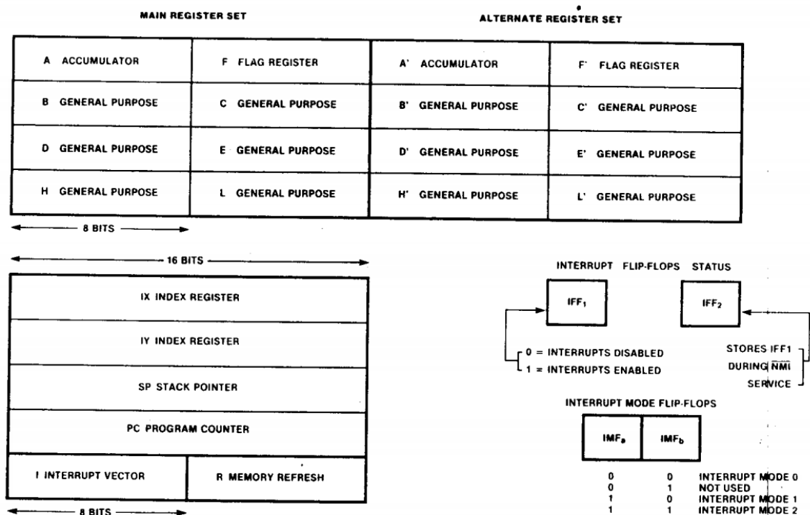
FIGURA 3-5 - REGISTRI DELLA CPU Z80 [19]
