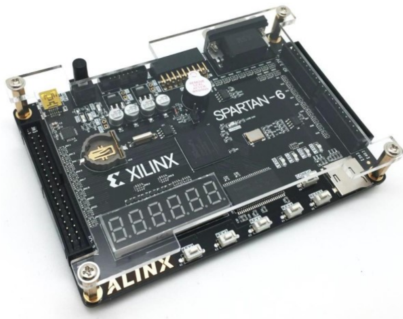
FIGURA 2-3 - SCHEDA DI SVILUPPO AX309
