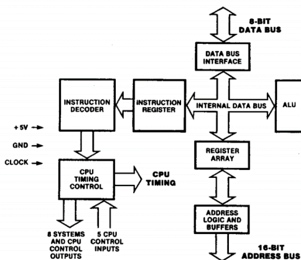
FIGURA 3-4 - DIAGRAMMA A BLOCCHI DELLO Z80 [19]
