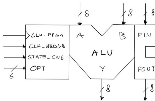
FIGURA 3-37 - SCHEMA DELL'ALU
