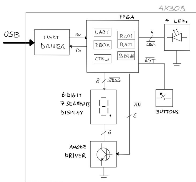
FIGURA 4-1 - SCHEMA DELLE UNITÀ USATE ALL'INTERNO DELLA SCHEDA AX309
