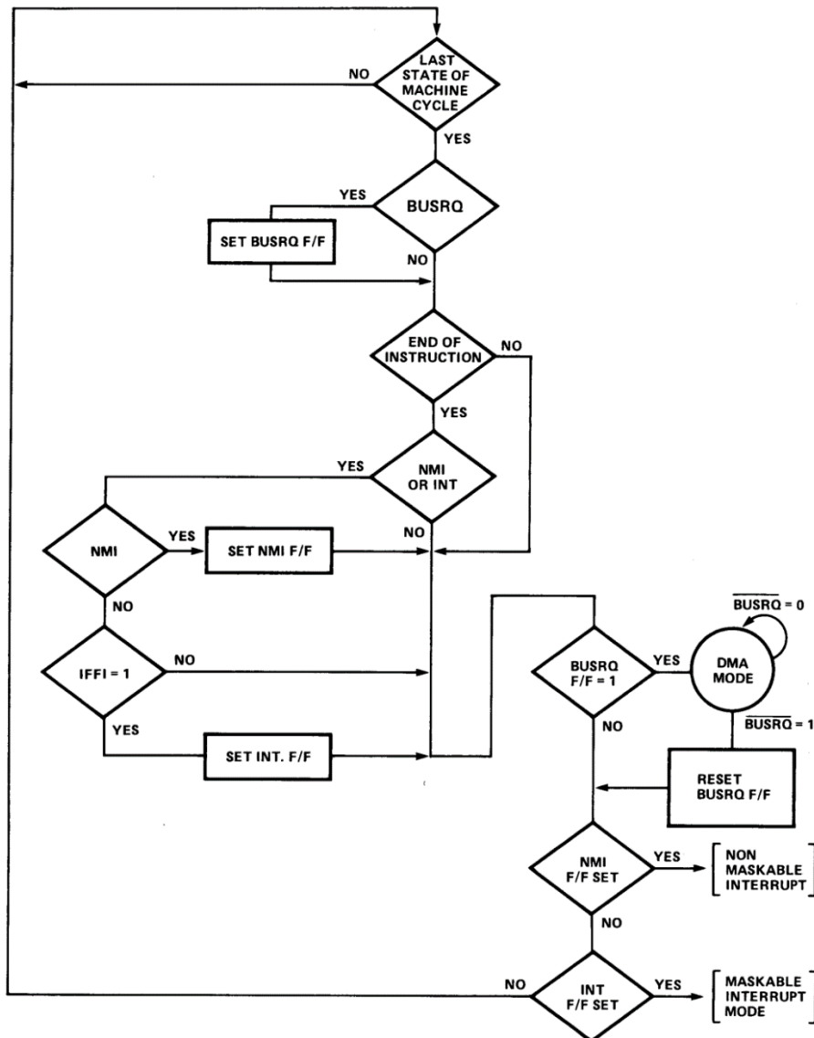
FIGURA 3-6 - DIAGRAMMA DI FLUSSO DELLA GESTIONE DEGLI INTERRUPT [24]
