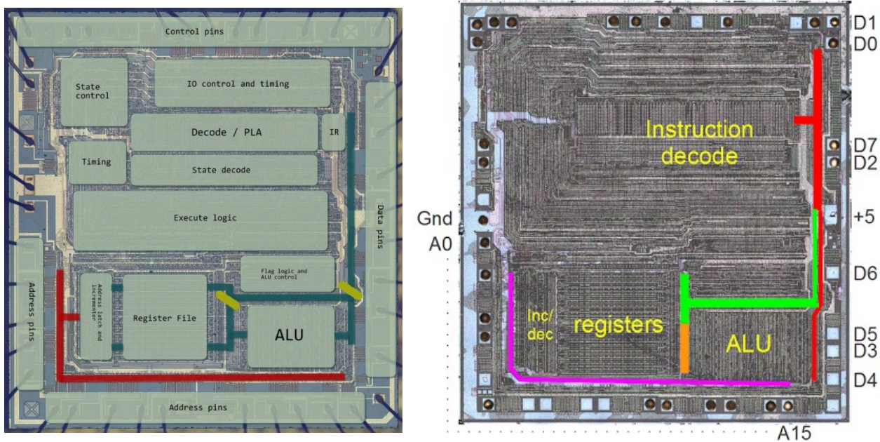
FIGURA 3-11 - DIE DELLO Z80 CON LE UNITÀ OPERATIVE [26]. ACCANTO, I DATA BUS INTERNI: IN ROSSO, VERDE E ARANCIO LE TRE SEZIONI DEL BUS A 8 BIT. IN FUCSIA, IL BUS INDIRIZZI A 16 BIT [28]
