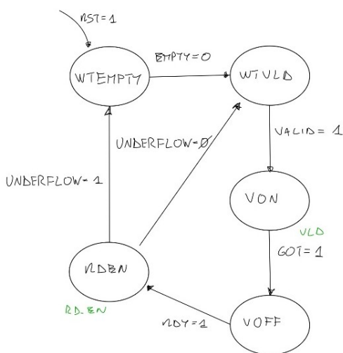
FIGURA 4-5 - DIAGRAMMA DI STATO DI CHAR_FEEDER_FIFO
