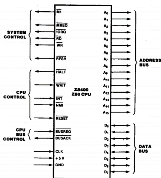
FIGURA 3-3 - PINOUT DELLO Z80 [19]
