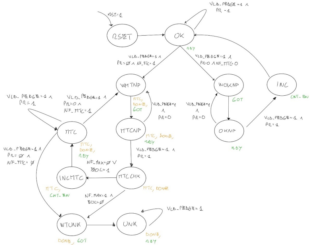
FIGURA 4-8 - DIAGRAMMA DI STATO DI FIELD_RECOGNIZER
