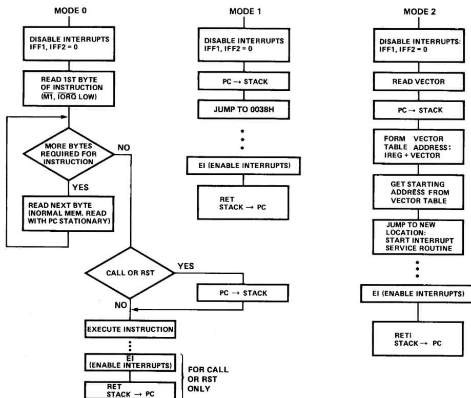
FIGURA 3-7 - SEQUENZE DI SERVIZIO DI UN INTERRUPT MASCHERABILE [24]
