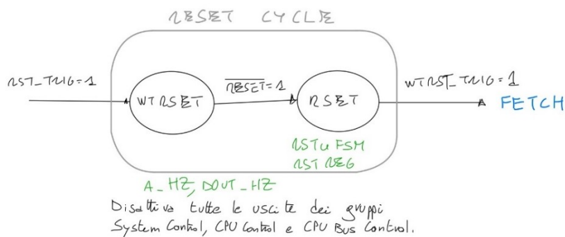
FIGURA 3-28 - DIAGRAMMA DI STATO DEL CICLO RESET CYCLE
