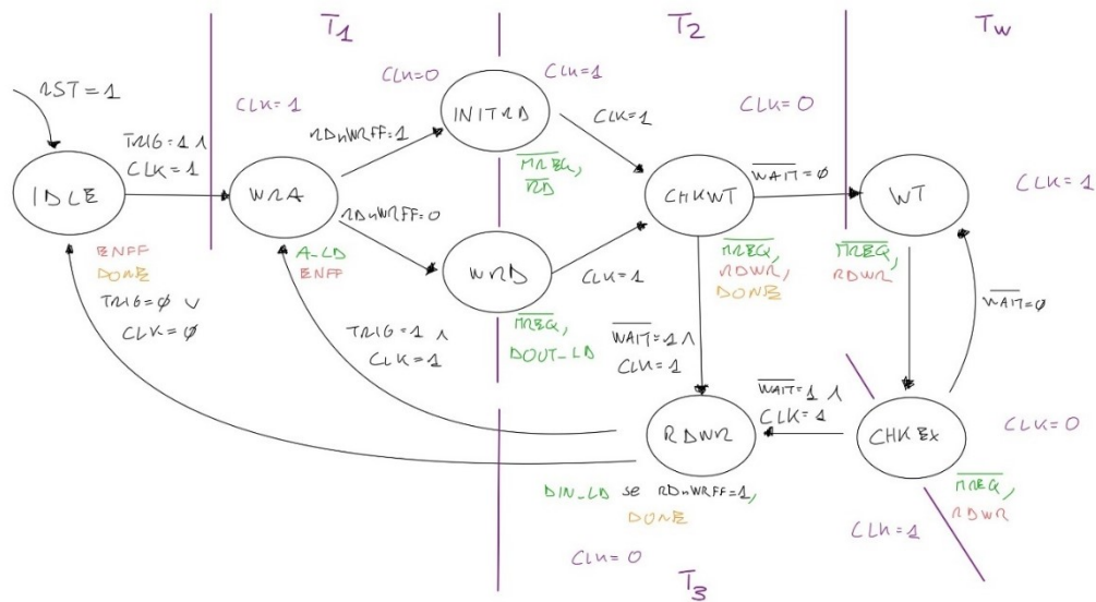
FIGURA 3-32 - DIGRAMMA DI STATO DELLA UFSM MEMRDWR
