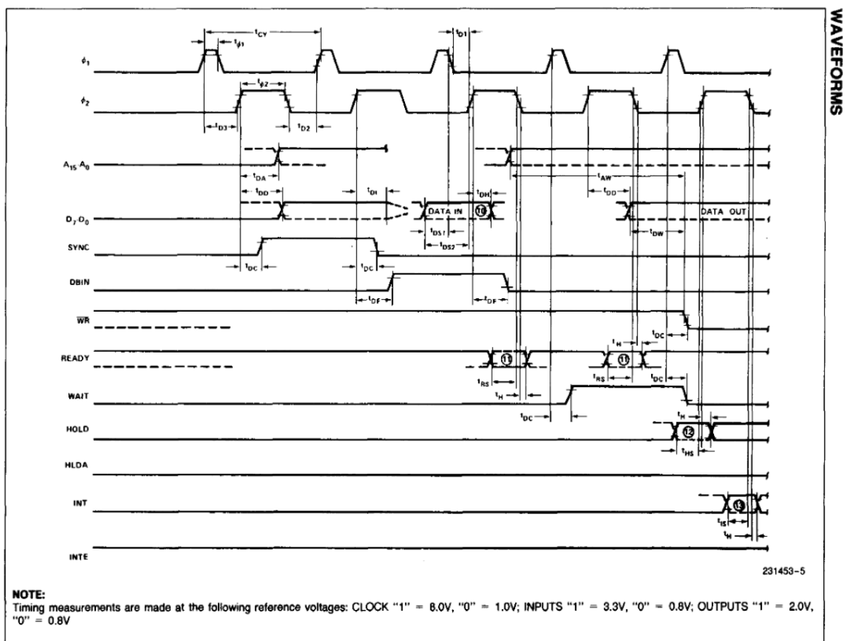
FIGURA 3-2 - FORME D'ONDA DEGLI INGRESSI E DELLE USCITE DELL'INTEL 8080° [18]
