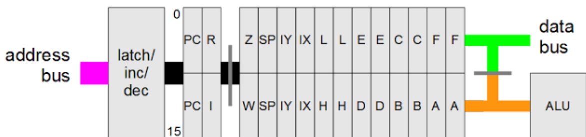
FIGURA 3-15 - STRUTTURA DEI REGISTRI DELLO Z80 [29]
