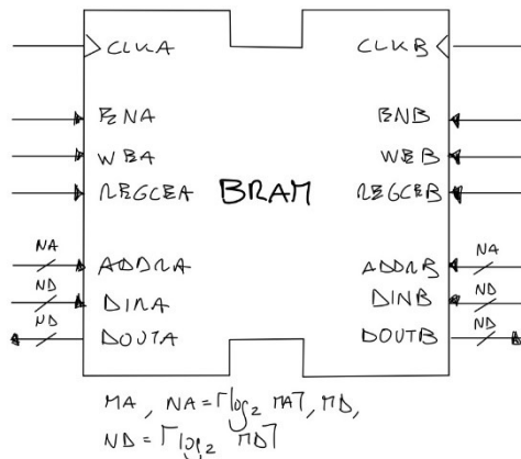
FIGURA 4-3 - SCHEMA DI UNA BRAM GENERICA
