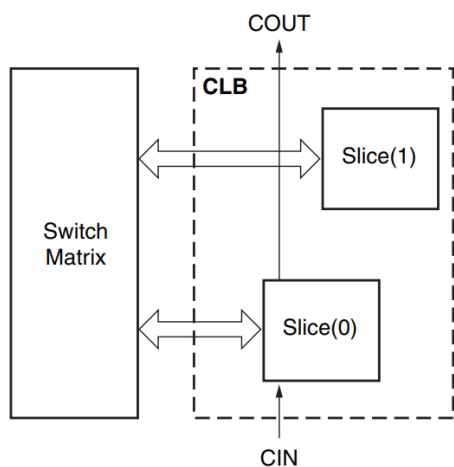
FIGURA 2-4 – DISPOSIZIONE DELLE SLICES ALL'INTERNO DI UN CLB [9]
