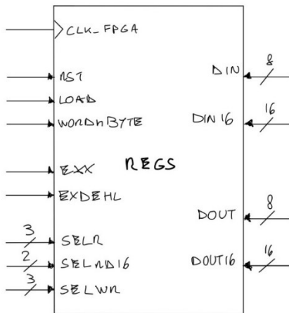
FIGURA 3-39 - SCHEMA DELL'ENTITY REGS
